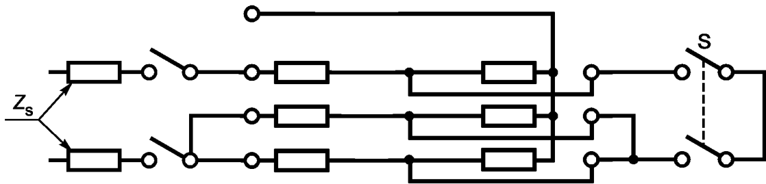
Рисунок 1 — Трансформатор со схемой соединения обмоток Y_n/D
