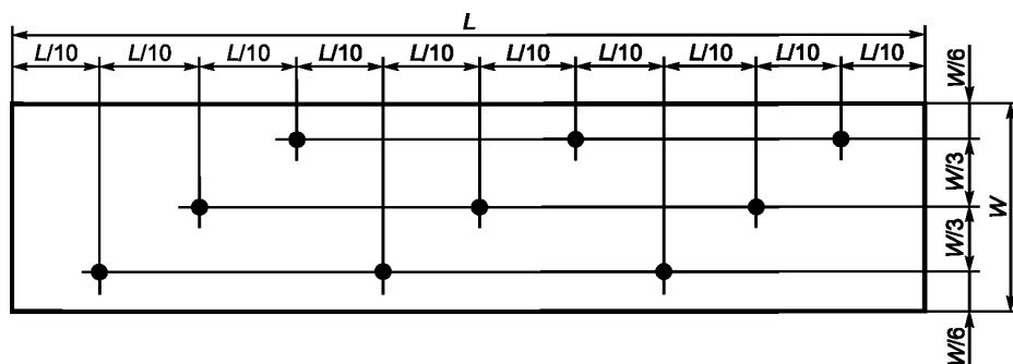
L — длина платформы; W — ширина платформы
