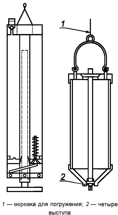
Рисунок 6 — Стержневая желонка закрытого типа
