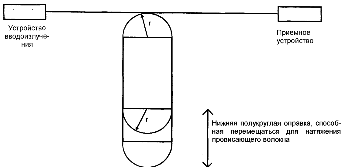
Рисунок 3 – Размещение волокна по умолчанию для измерения \lambda_c
