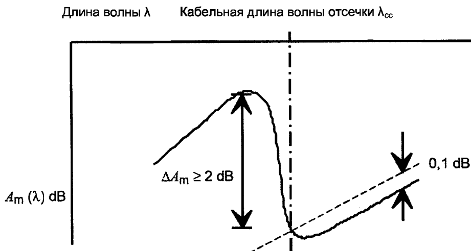
Рисунок 6 – Измерение длины волны отсечки при использовании методики эталонного многомодового волокна
