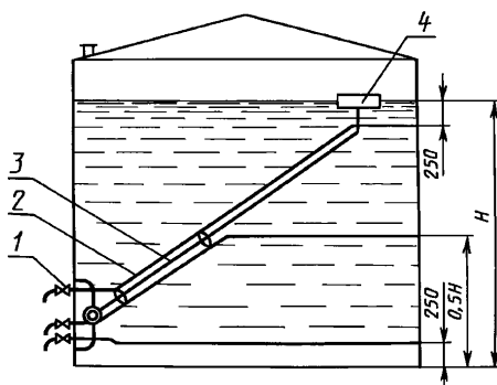
1 — кран; 2 — пробозаборные трубки; 3 — несущий рычаг; 4 — поплавок
