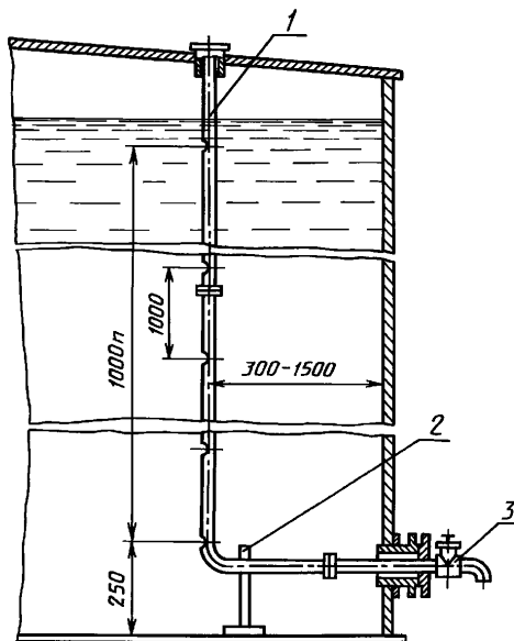
1 — перфорированная заборная трубка; 2 — опорная стойка; 3 — кран
