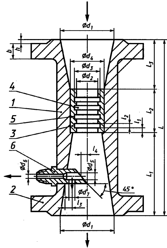
Диспергатор
