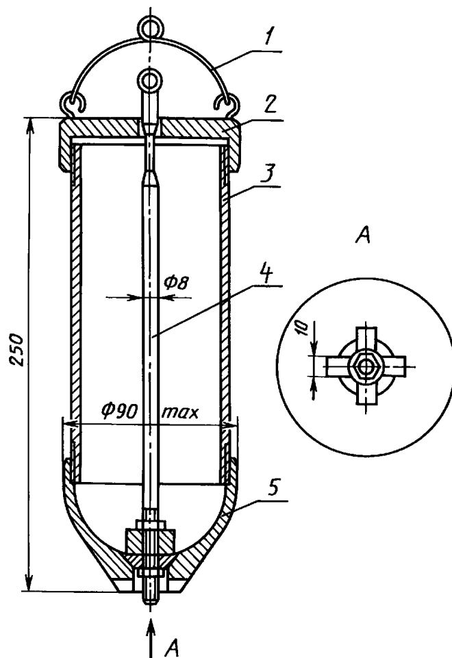
1 — скоба; 2 — крышка с клапаном; 3 — корпус; 4 — шток с клапаном; 5 — днище
