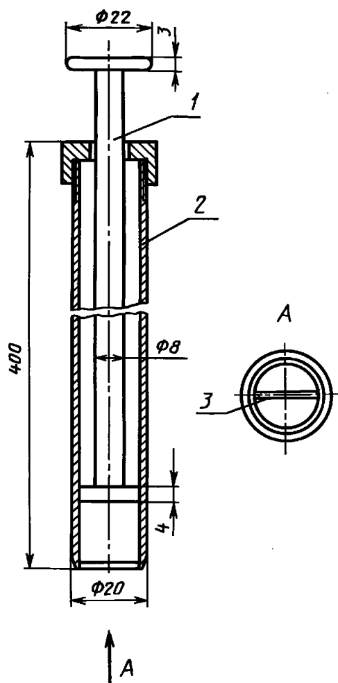
Поршневой щуп
