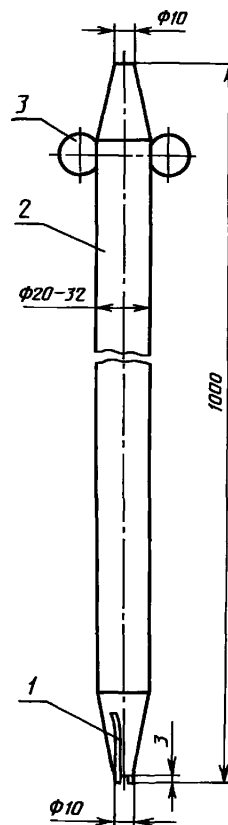
Пробоотборная трубка
