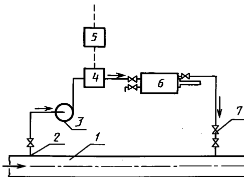
1 — трубопровод; 2 — пробозаборное устройство; 3 — насос; 4 — запорное устройство; 5 — регулятор; 6 — пробоотборник; 7 — обратный клапан
