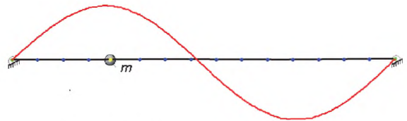
Форма № 2 (частота f = 29,3 Гц)
