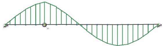
Эпюра усилий/напряжений для формы № 2
