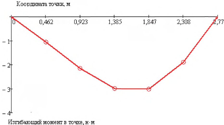
Рисунок А.7 – График изменения изгибающих моментов \{S\} в трубопроводе под действием вибрационной нагрузки
