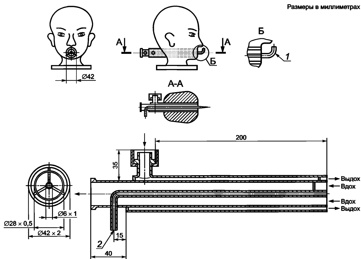
Рисунок 2 — Муляж головы человека (голова Шеффилда)
