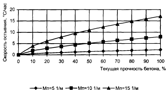
Рисунок 1. Максимальные скорости остывания бетона
