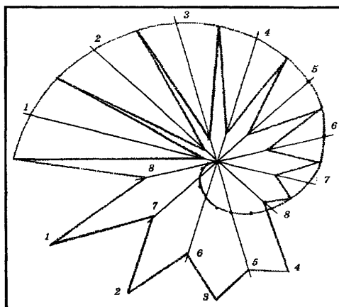
Рис.2. Возможное размещение датчиков фотонного излучения в СЗЗ по спирали Архимеда (на пересечении кривой с лучами) и многолучевой звездой в вершинах и основаниях лучей [8]
