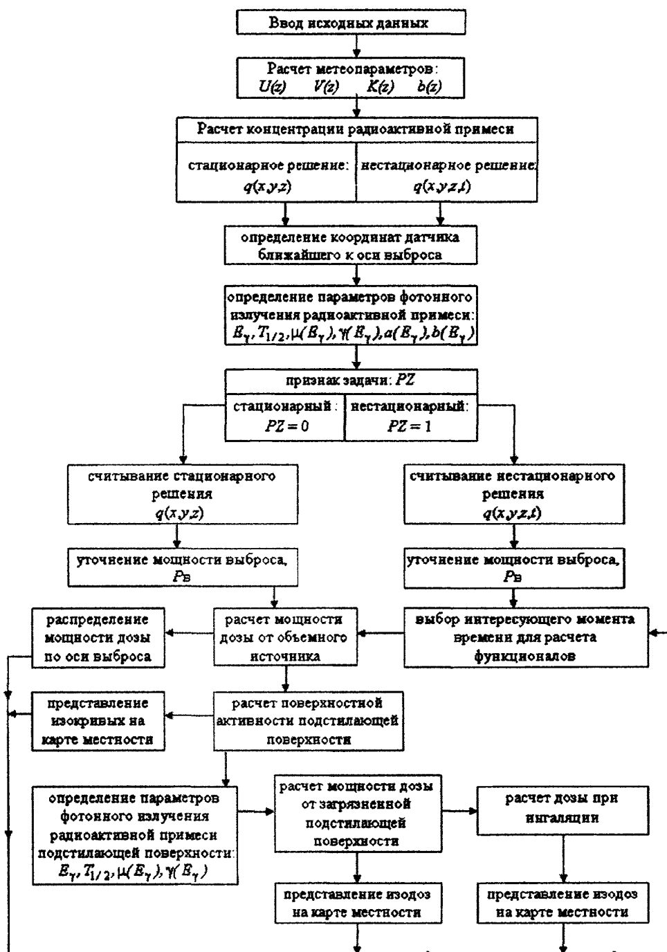
Рис. 2. Алгоритм расчета загрязнения окружающей среды и дозовых нагрузок на персонал и население
