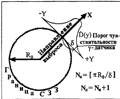
Рис.1. Иллюстрация выбора оптимального количества датчиков АСКРО
