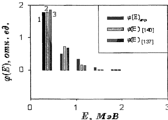
Рис.1. Гистограммы спектров фотонного излучения:
