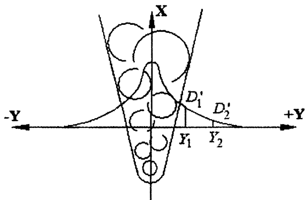
Рис.1. Оценка величины мощности выброса радиоактивной примеси в атмосферу с учетом фоновых значений мощности дозы естественного или техногенного происхождения
