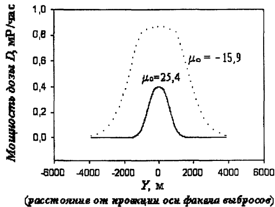
Рис.2. Распределение мощности дозы в направлении, перпендикулярном оси факела выбросов при X = 2750 м при устойчивом \mu_0 = 25,4 и неустойчивом \mu_0 = -15,8 состояниях атмосферы [5]
