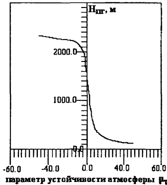
Рис.1. Зависимость высоты пограничного слоя атмосферы от состояния ее устойчивости, характеризуемой параметром \mu_0
