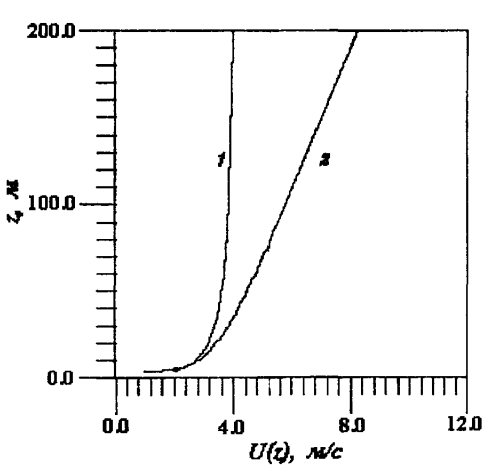
Рис. 1. Зависимость скорости приземного ветра U(z) от высоты от подстилающей поверхности (модель приземного слоя атмосферы): 1 – неустойчивое состояние ( L = -18 , v_* = 0,32 м/с), 2 – устойчивое состояние ( L = 30 , v_* = 0,26 м/с)
