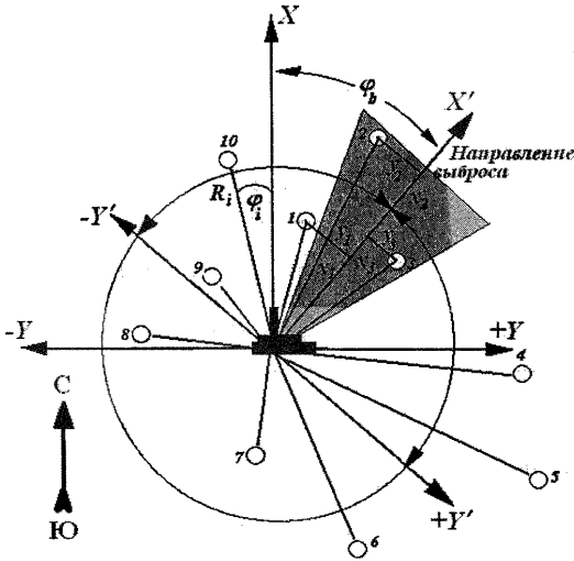
Рис.1. Геометрия определения координат и номера датчика, ближайшего к оси выброса радиоактивной примеси: 1–10 – детекторы фотонного излучения постов контроля АСКРО; (X, Y) – жесткая система координат; (X', Y') – локальная система координат
