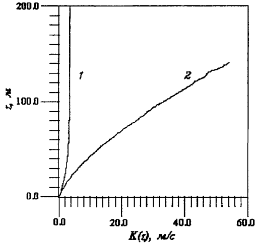
Рис.2. Зависимость коэффициента турбулентной диффузии K(z) от высоты от подстилающей поверхности при различных состояниях устойчивости атмосферы: 1 – неустойчивое состояние ( L = -18 ), 2 – устойчивое состояние ( L = 30 )
