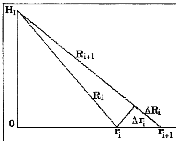
Рис.3. Определение приращения радиуса-вектора R_i и его последующего значения по предыдущему
