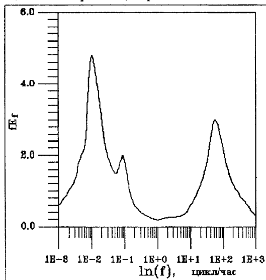
Рис.1. Спектр скорости ветра в приземном слое атмосферы [2]
