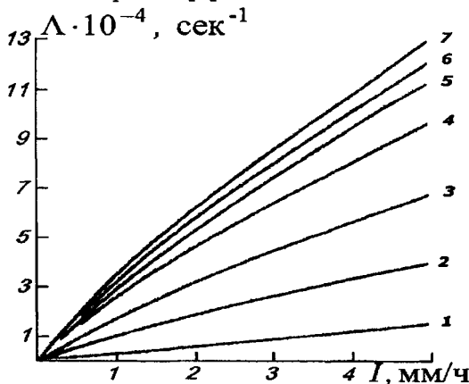
Рис. 1. Коэффициенты вымывания частиц единичной плотности из подоблачного слоя атмосферы в зависимости от интенсивности дождя I для различных значений a_2p (Chamberlain, 1953.) [4]: 1 – 4 \text{ мкм}^2 \cdot \text{г}/\text{см}^3 ; 2 – 7,8 \text{ мкм}^2 \cdot \text{г}/\text{см}^3 ; 3 – 16 \text{ мкм}^2 \cdot \text{г}/\text{см}^3 ; 4 – 41 \text{ мкм}^2 \cdot \text{г}/\text{см}^3 ; 5 – 81 \text{ мкм}^2 \cdot \text{г}/\text{см}^3 ; 6 – 169 \text{ мкм}^2 \cdot \text{г}/\text{см}^3 ; 7 – 400 \text{ мкм}^2 \cdot \text{г}/\text{см}^3
