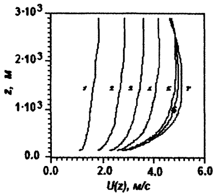
Рис.2. Зависимость продольной составляющей скорости ветра U(z) от высоты при различном состоянии устойчивости атмосферы (1-7) в модели пограничного слоя атмосферы
