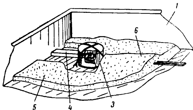
Рис. 3. Замоноличивание электропроводки в стенную шлакобетонную панель, изготовляемую в горизонтальной форме
