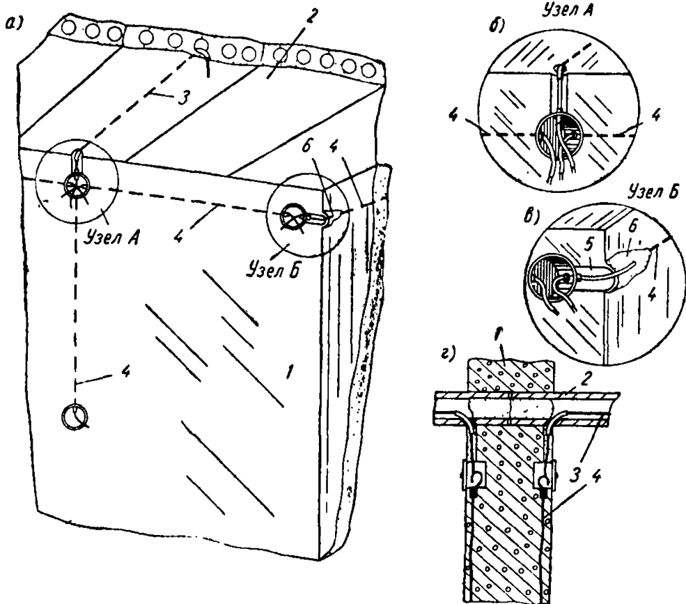
Рис. 15. Узлы сопряжения электропроводок, замоноличенных в стеновые панели при изготовлении на заводе (случай, когда к потолочным светильникам провода прокладываются в пустотах панелей перекрытия)
