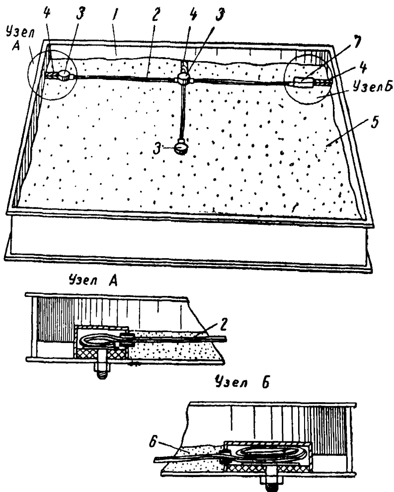
Рис. 2. Замоноличивание электропроводки в стенную шлакобетонную панель, изготавливаемую в горизонтальной форме
