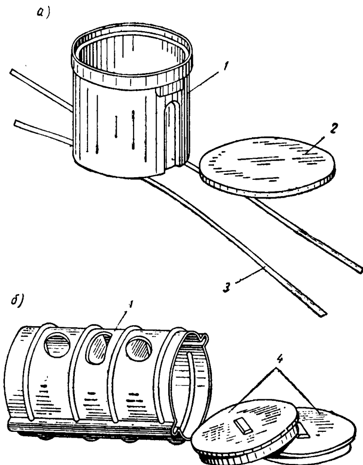
Рис. 1. Коробки для замоноличенных электропроводок а — пластмассовая коробка, применяемая в прокатных железобетонных панелях заводом железобетонных конструкций № 6 Главмостроя (изготавливается заводом ЭТИ Главмостроя); б — металлическая двухсторонняя коробка, применяемая при изготовлении панелей в кассетных установках домостроительным комбинатом № 2 Главленинградстроя (изготавливается заводом ЭТИ треста Электромонтаж-55 Главленинградстроя); 1 — корпус коробки; 2 — крышка с резьбой; 3 — проволока металлическая; 4 — крышка
