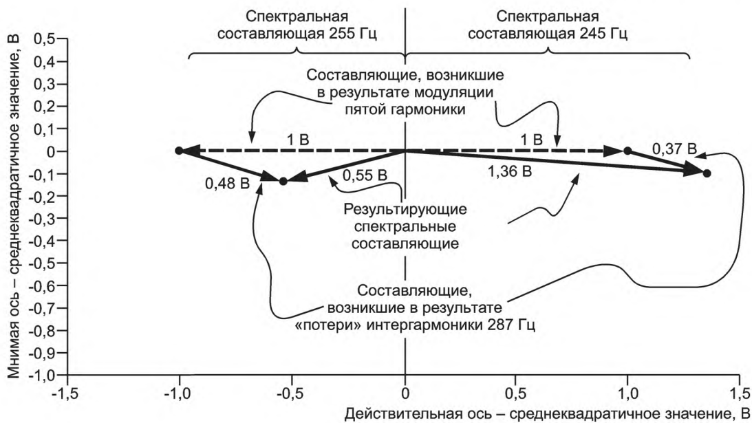
Рисунок С.7 — Векторы спектральных составляющих на частотах 245 и 255 Гц
