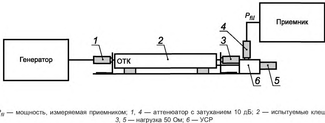
Рисунок В.9 — Установка для измерения коэффициента развязки DR
