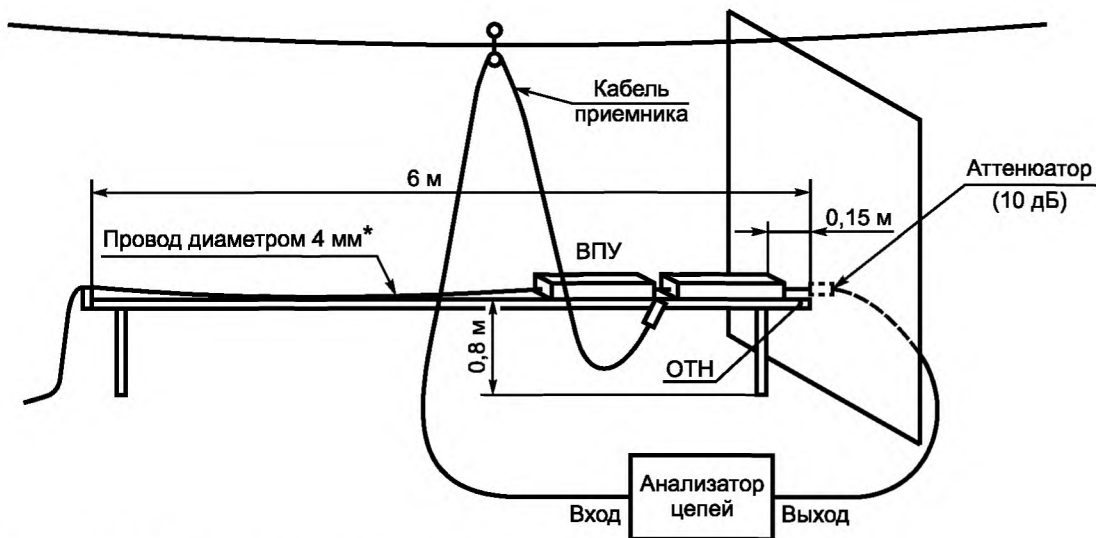
а) Измерение мощности генератора
