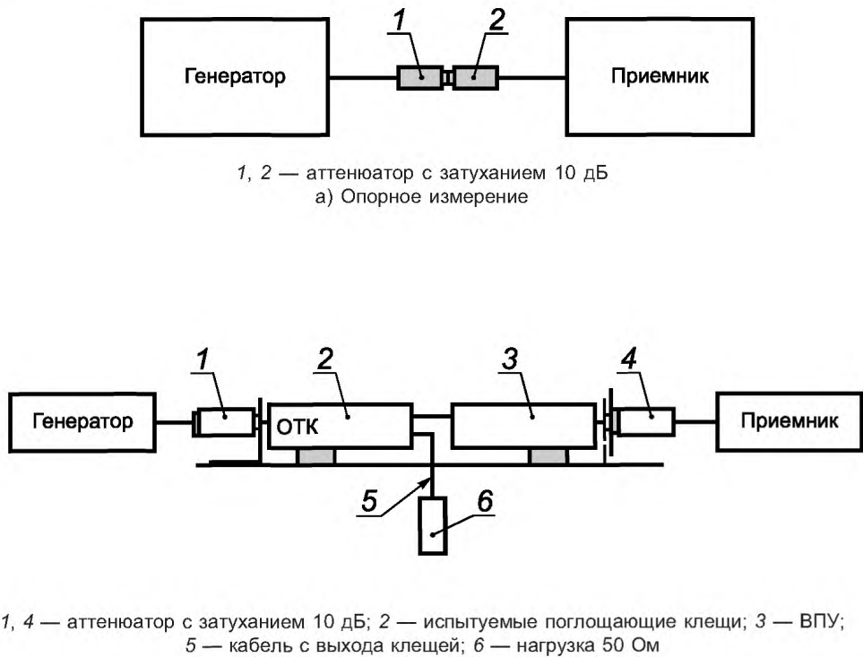
Рисунок В.8 — Установка для измерения коэффициента развязки DF
