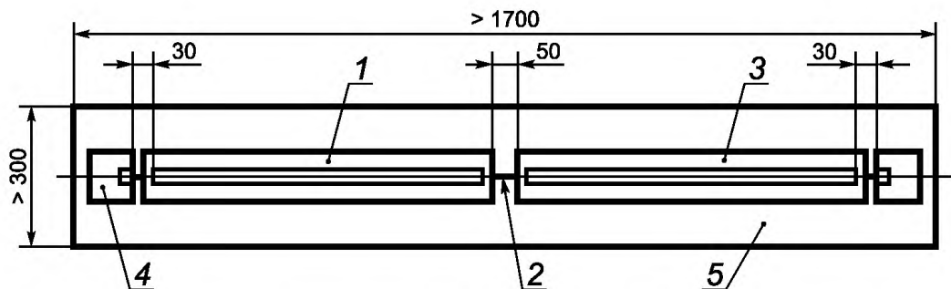
1 — поглощающие клещи; 2 — провод диаметром 4 мм; 3 — ВПУ; 4 — электрическая связь с пластиной заземления; 5 — металлическая пластина заземления
