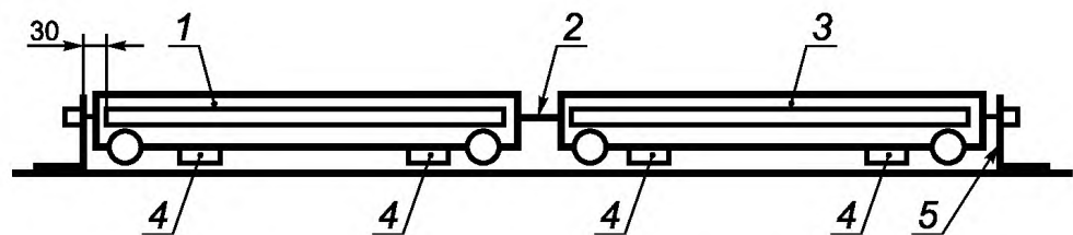
1 — поглощающие клещи; 2 — провод диаметром 4 мм; 3 — ВПУ; 4 — непроводящая прокладка для регулировки высоты клещей над пластиной заземления; 5 — электрическая связь с пластиной заземления
