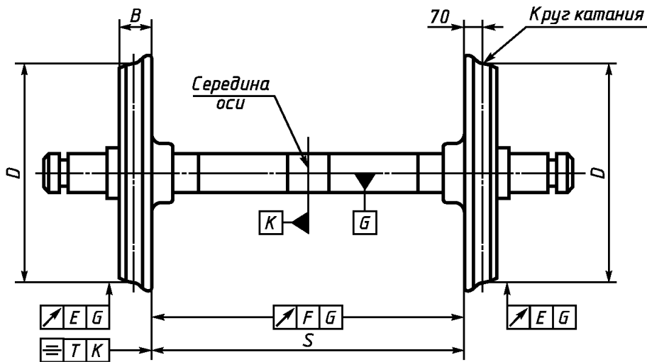
S — расстояние между внутренними торцами (гранями) ободьев колес; B — ширина обода колеса; K — плоскость симметрии оси; T — допуск симметричности размера S ; D — диаметр колес по кругу катания; E — допуск радиального биения круга катания колеса; F — допуск торцевого биения внутреннего торца обода колеса; G — ось центров Рисунок 1 — Колесная пара в сборе (неприводная)
