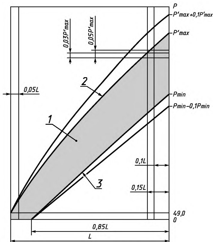
Рисунок 3 — Шаблон-диаграмма запрессовки
