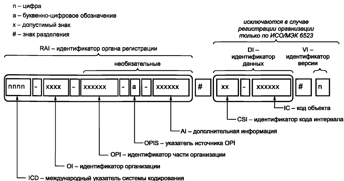
Рисунок 1 — Структура идентификатора IRDI
