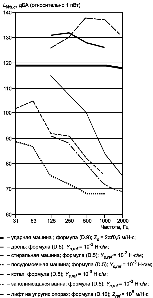
Рисунок D.4 — Зависимости от частоты уровня характеристической мощности некоторых источников структурного шума, определенные с помощью формул (D.5), (D.9) и (D.10) на основании результатов измерений силы или скорости вибрации [11], [17], [18]
