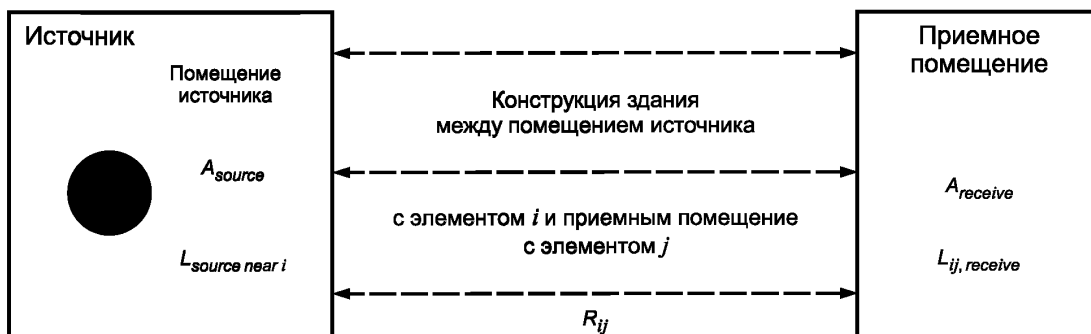
Рисунок 2 — Звукопередача воздушного шума от источника по пути ij
