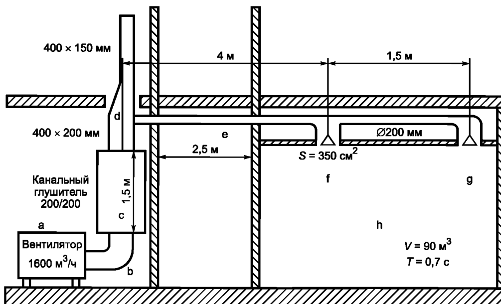
Рисунок I.1 — Пример вентиляционной системы
