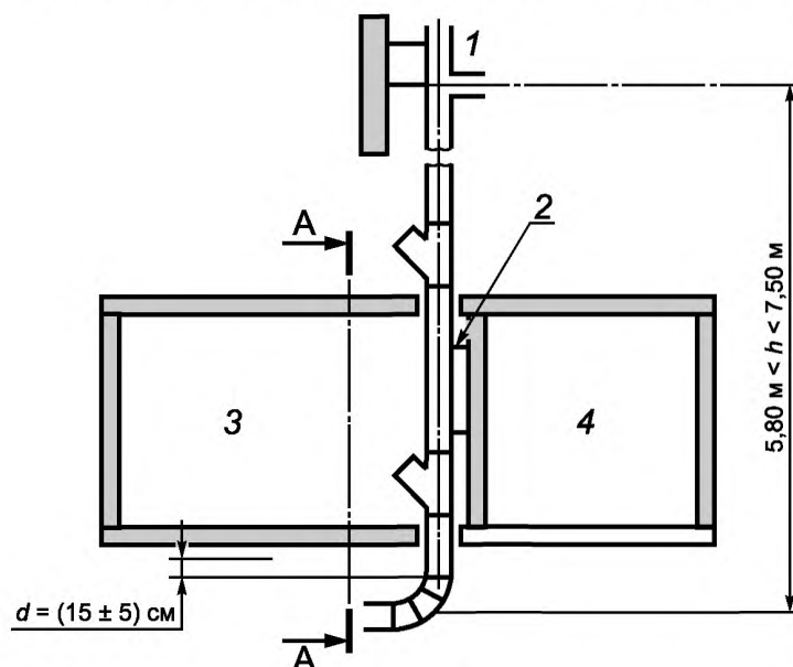
Рисунок D.2 — Стандартная испытательная установка для оборудования системы канализации по [38]
