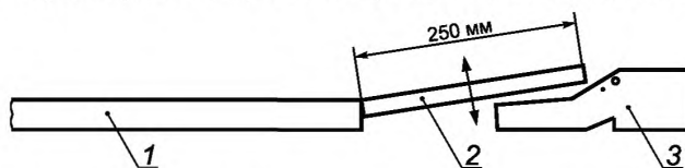
1 — стапельная платформа; 2 — выступающая защитная накладка; 3 — нога
