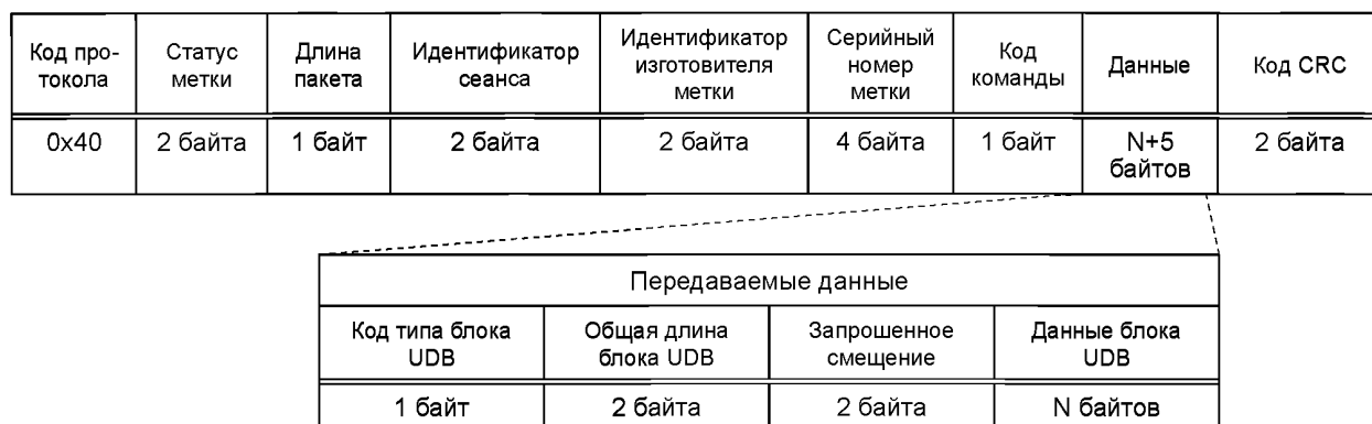
Рисунок 11 — Ответ радиочастотной метки на запрос дополнительной информации с помощью частной команды «Read UDB»
