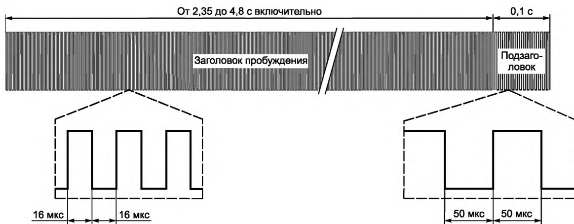
Рисунок 1 — Сигнал пробуждения «Wake Up»
