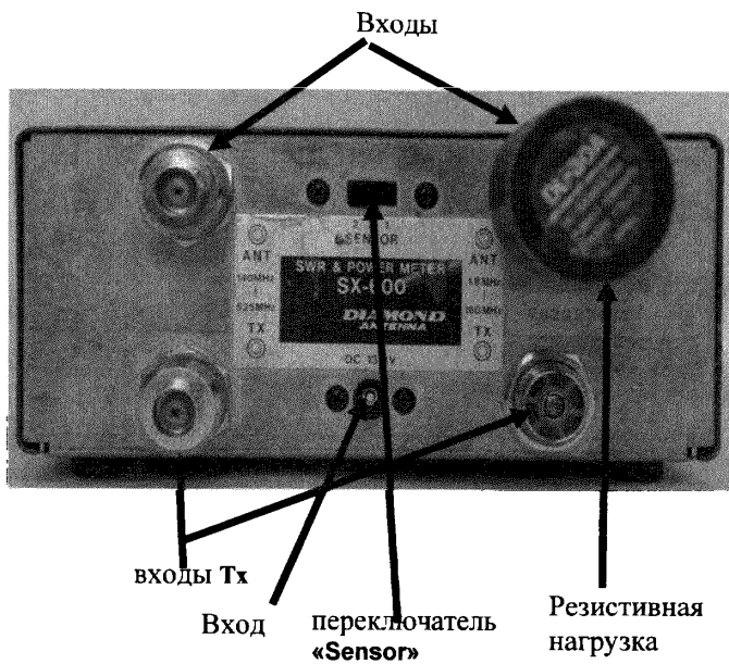
Рис. 6 Задняя панель КСВ-метра DIAMOND SX-600
