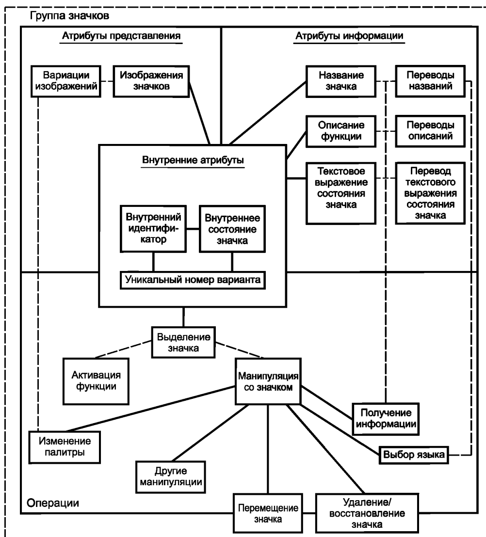
Рисунок 2 — Детальная схема определения доступности графических значков
