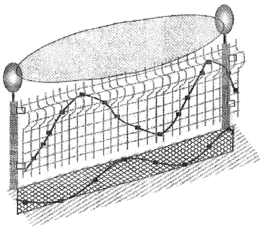
Рисунок 121 – Установка извещателя «Рубеж» на стальной сварной сетке
