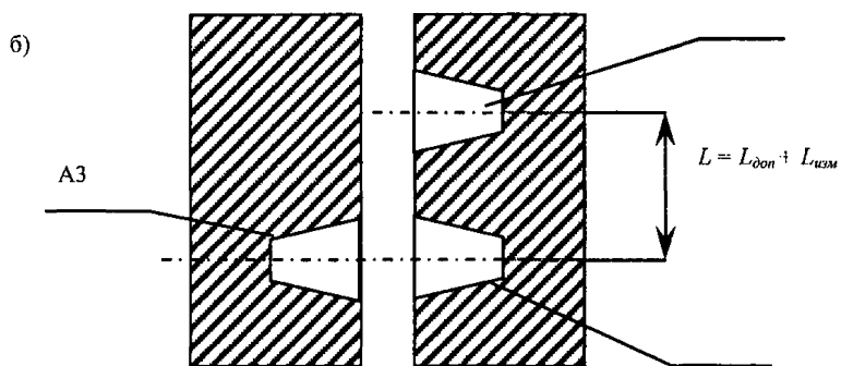
Рисунок 10 – Схема размещения мест монтажа извещателя и ДВМП
