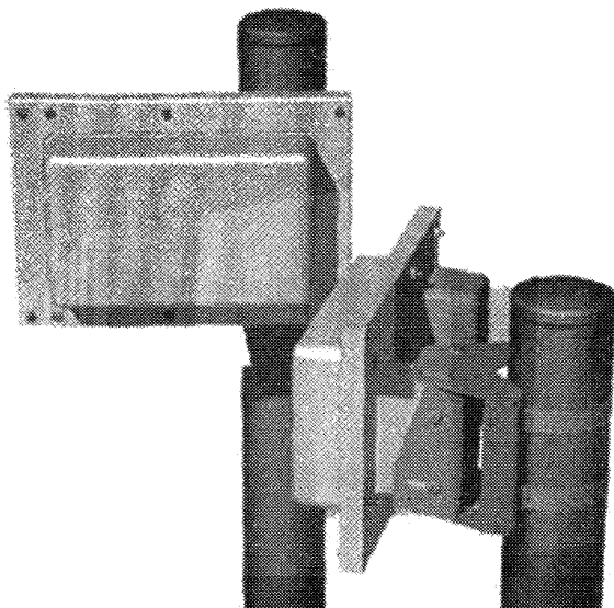
Рисунок 91 - Извещатель «Линар-200»
