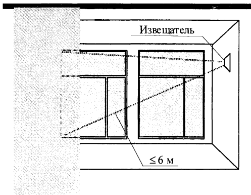
Рисунок 15 – Между стеклом и жалюзи
