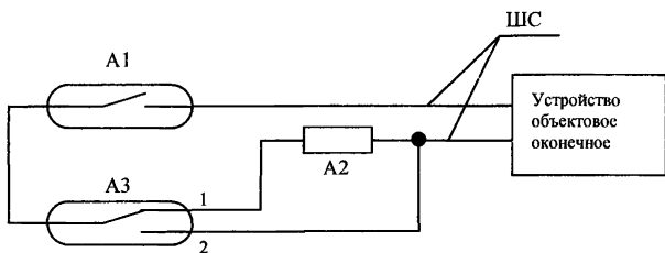
Рисунок 9 – Схема защиты магнитоcontactного извещателя от саботажа
