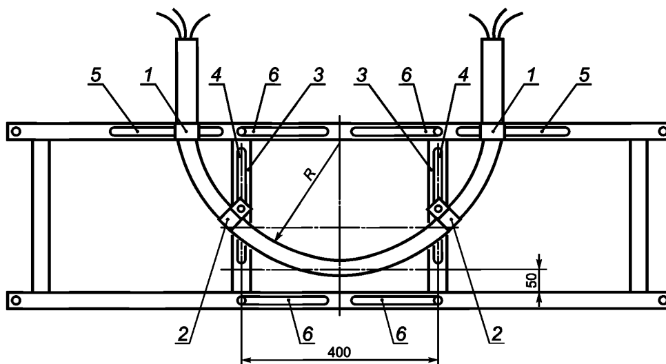
1 — U-образный хомут; 2 — P-образный хомут; 3 — регулируемый вертикальный элемент; 4 — прорезь для фиксации U-образного хомута; 5 — прорезь для фиксации P-образного хомута; 6 — прорезь для перемещения вертикального элемента; R — минимальный радиус изгиба кабеля
