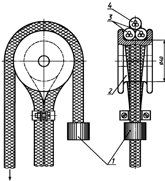
Рисунок 3 — Устройство для испытания на износостойкость
