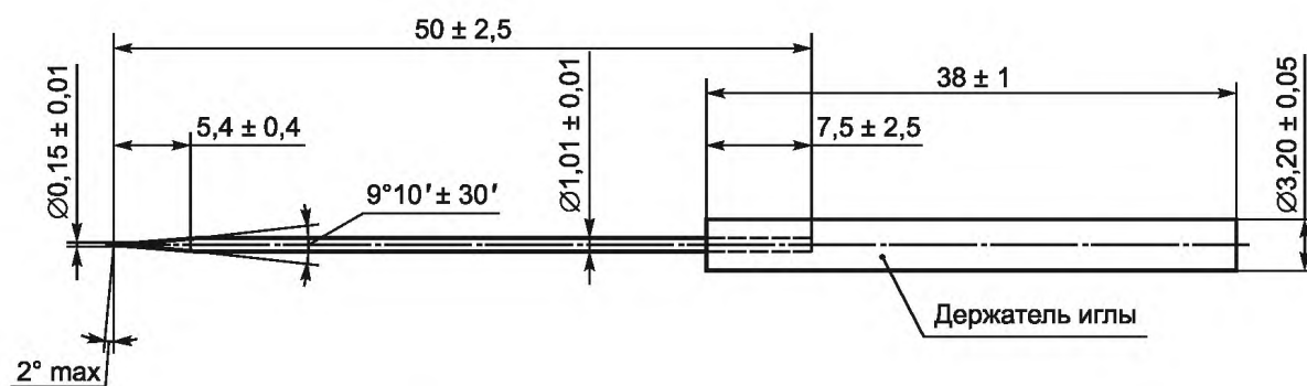
Рисунок А.2 — Пенетрационная игла
