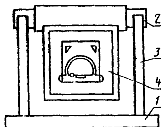
1 — плита; 2 — контрольный валик; 3 — опоры; 4 — рамный уровень
