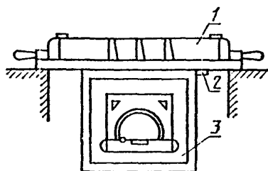
1 — поверочная плита; 2 — упорная планка; 3 — рамный уровень
