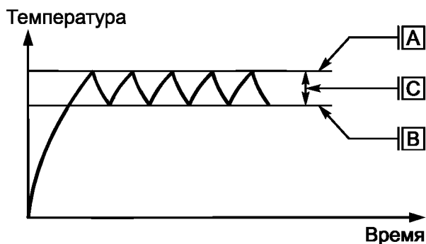
Рисунок ЕЕ.2 — Термоограничитель с самовозвратом
