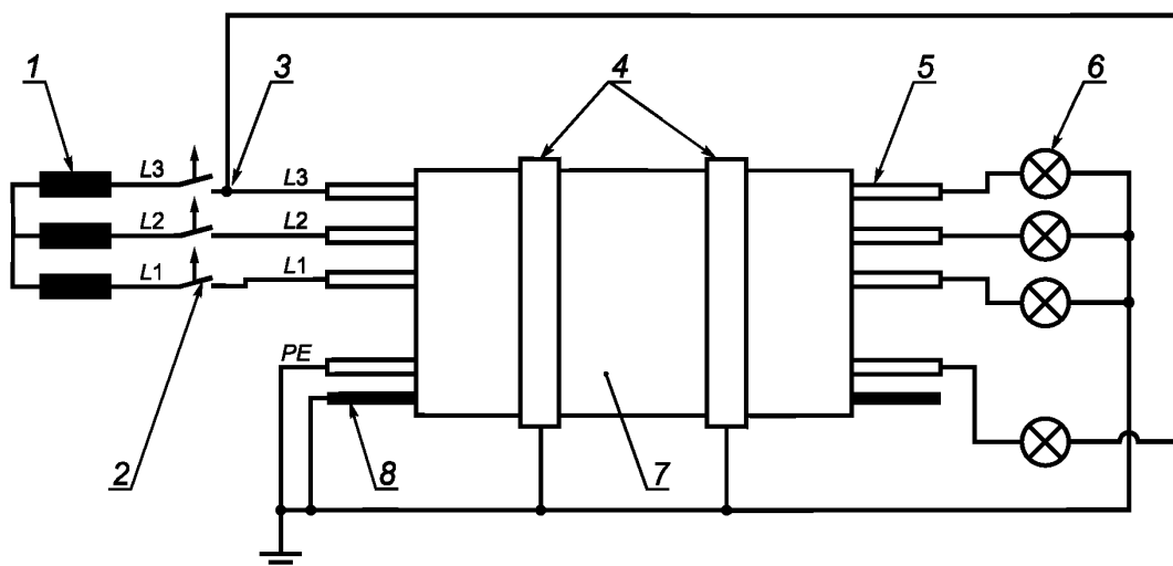
1 — трансформатор; 2 — плавкий предохранитель (2 А); 3 — подсоединение к линии L3 (или L1 , или L2 ); 4 — поддерживающие кольца; 5 — испытательная жила или группа жил; 6 — нагрузочный индикаторный прибор (например, лампа); 7 — образец; 8 — металлический экран (если имеется); L1 , L2 , L3 — линии испытываемых жил или групп жил ( L2 , L3 , если имеются); PE — жила заземления (если имеется)
