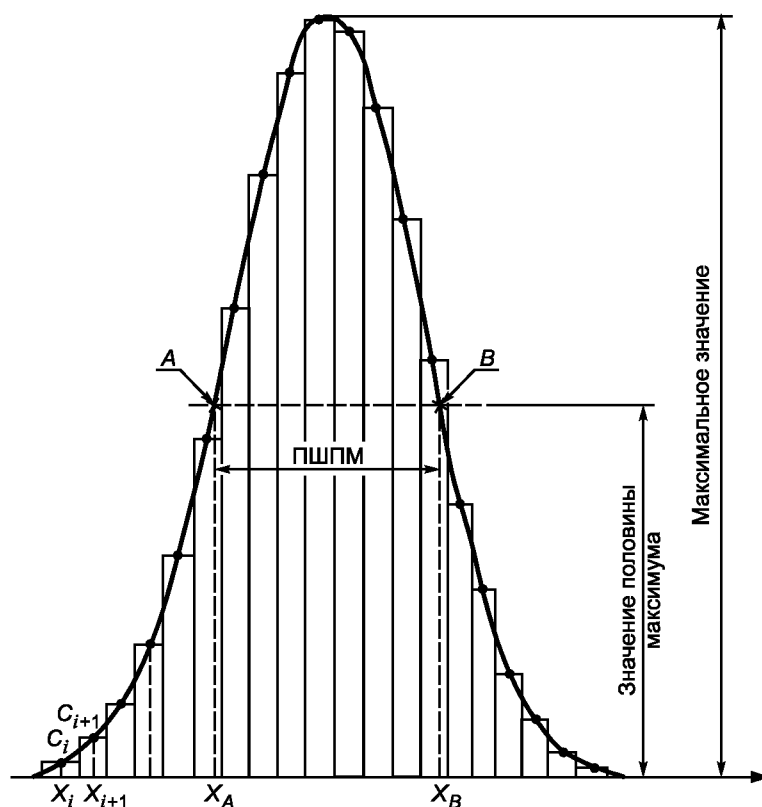
Рисунок 6 — Оценка ПШПМ
