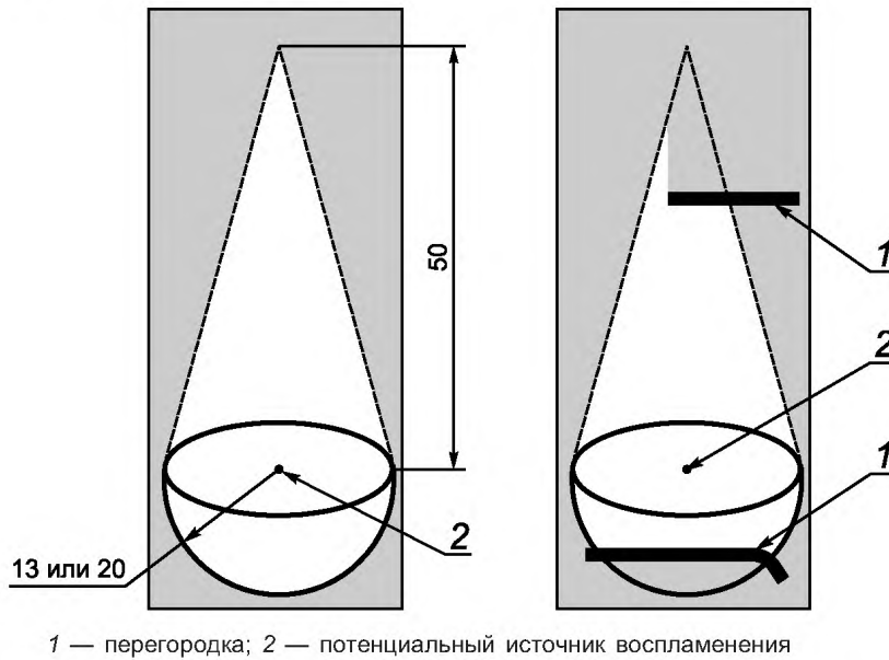
Рисунок 12 — Образец царпин для испытаний на взрывоопасность
