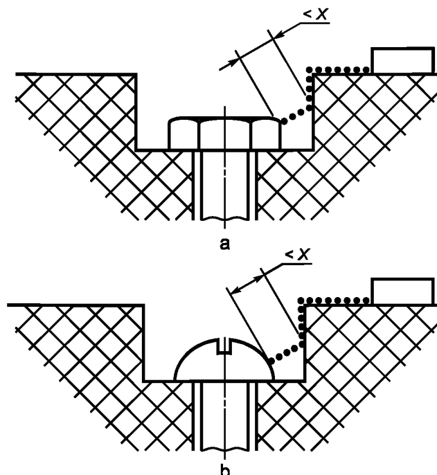
Рисунок E.8 — Промежуточная, несоединенная проводящая часть
