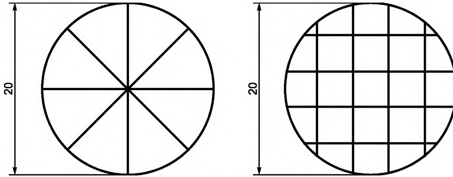
Рисунок 12 — Образец царпин для испытаний на взрывоопасность
