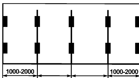
Рисунок В.3 — Размещение пяти пар опорных площадок
