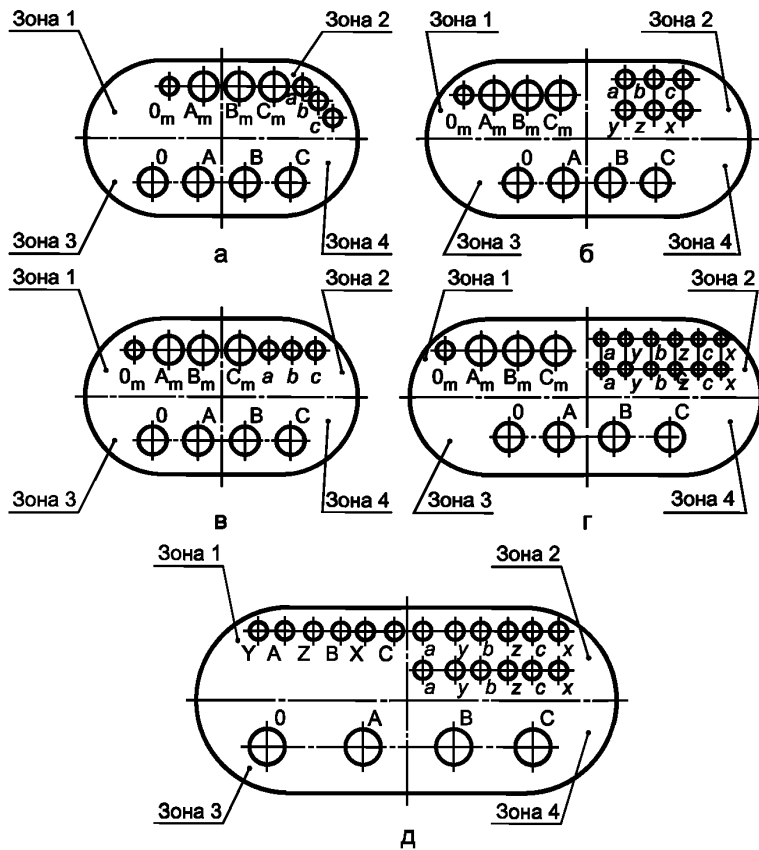
Рисунок 3 — Трехобмоточные трансформаторы
