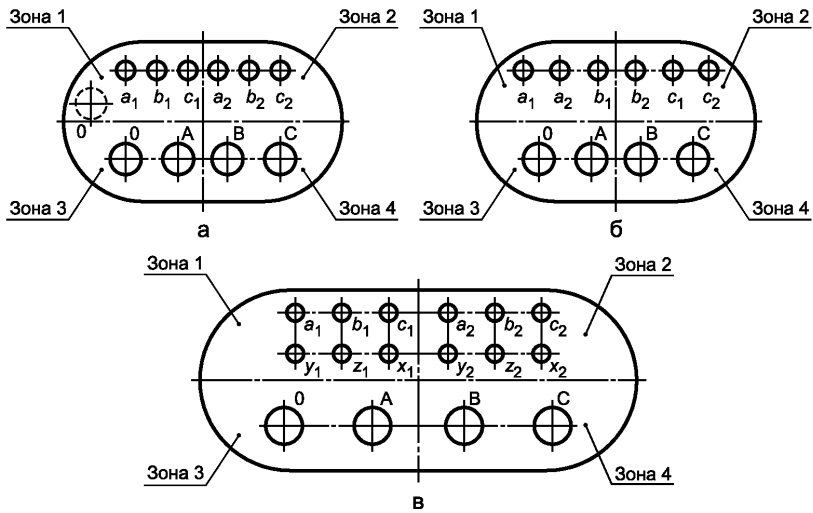
Рисунок 2 — Двухобмоточные трансформаторы с расщепленной обмоткой НН
