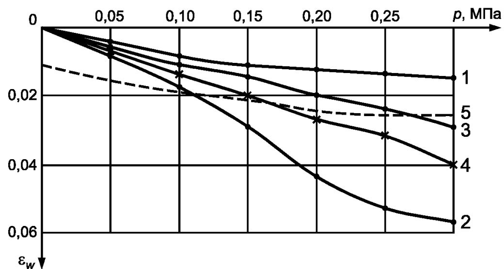
а) График зависимости относительного сжатия грунта при различной влажности от давления
