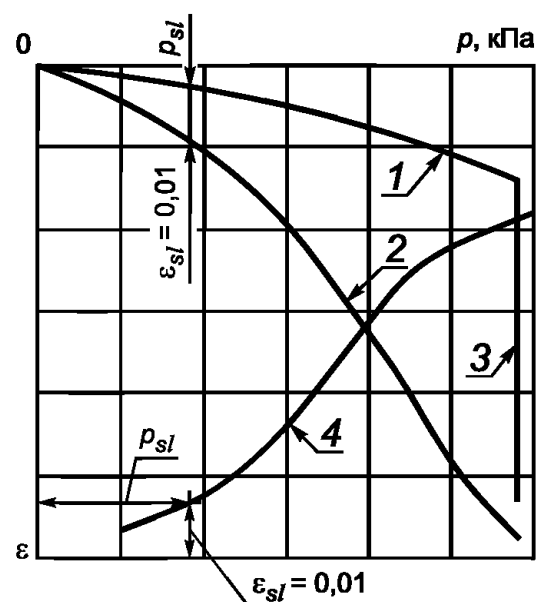
б) По схеме «двух кривых»
