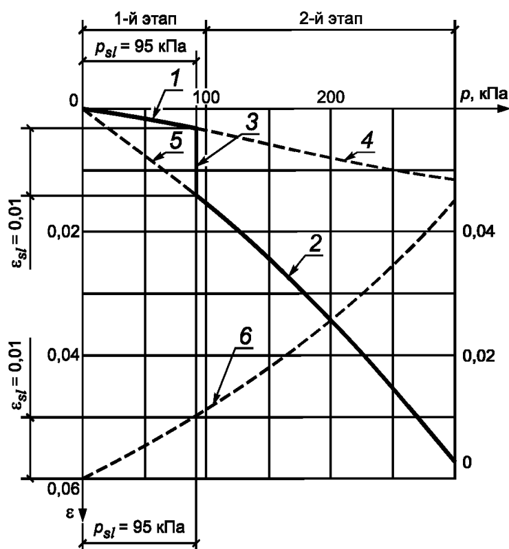
Рисунок В.1 — График испытания просадочного грунта ускоренным методом по «комбинированной схеме»
