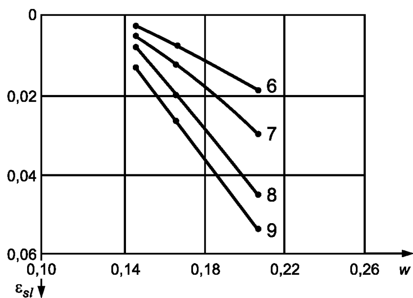
в) График зависимости относительной просадочности от влажности
