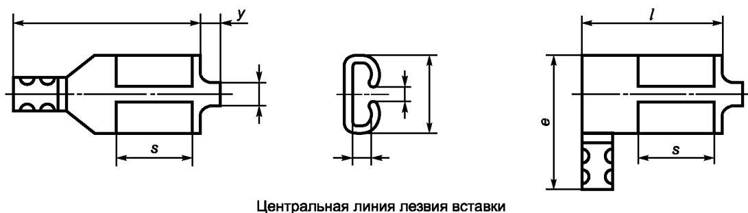
Центральная линия лезвия вставки
