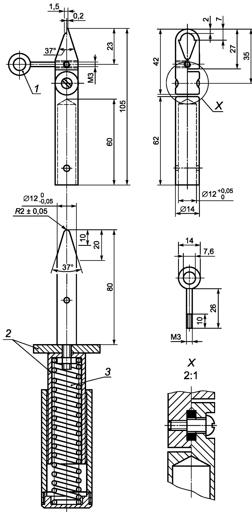
1 — петля; 2 — изолирующий материал; 3 — пружина диаметром 18 мм
