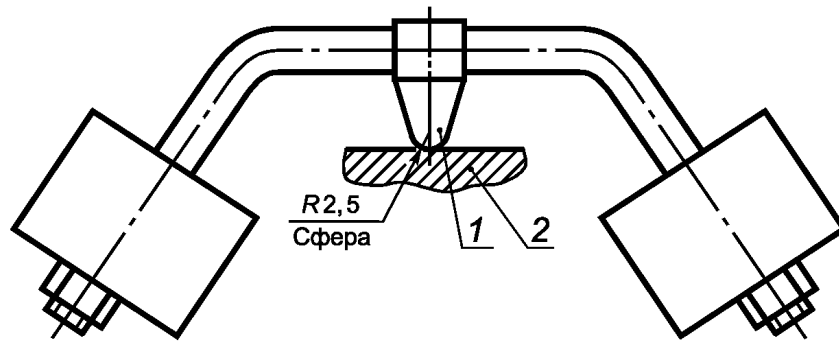
Рисунок 6 — Устройство для вдавливания шарика
