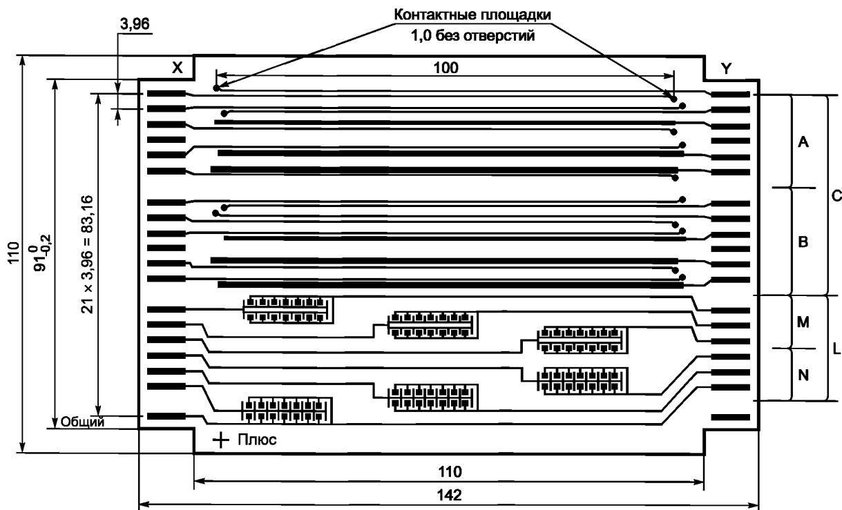
Рисунок Q.1 — Испытуемый образец
