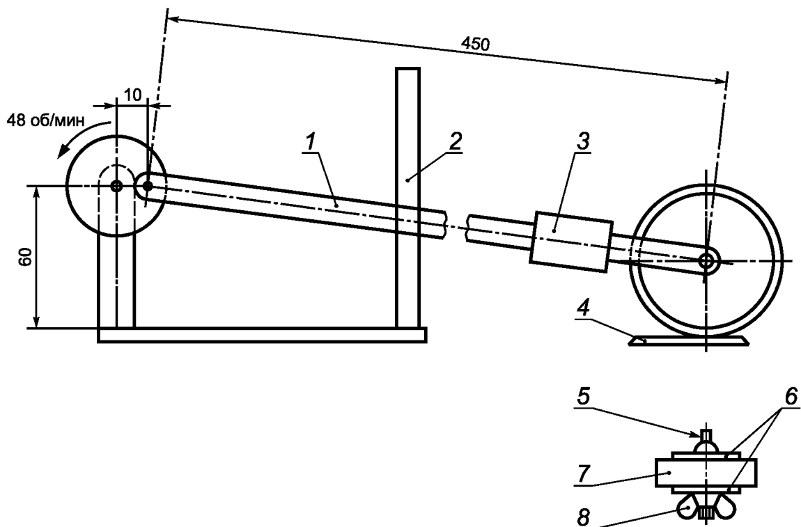
Рисунок 7 — Испытание горением
