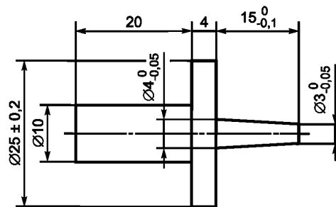
Рисунок 1 — Испытательный стержень
