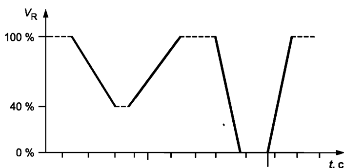
Рисунок Н.26.5.4.2 — Испытание изменения напряжения
