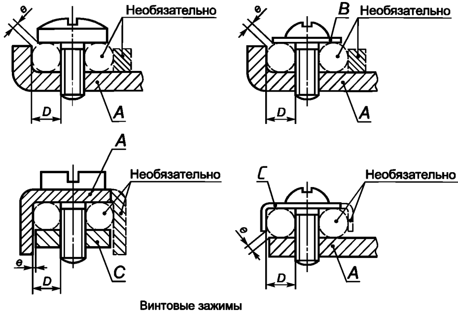
Винтовые зажимы
