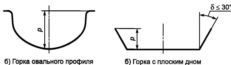
Рисунок 8 — Профили горки
