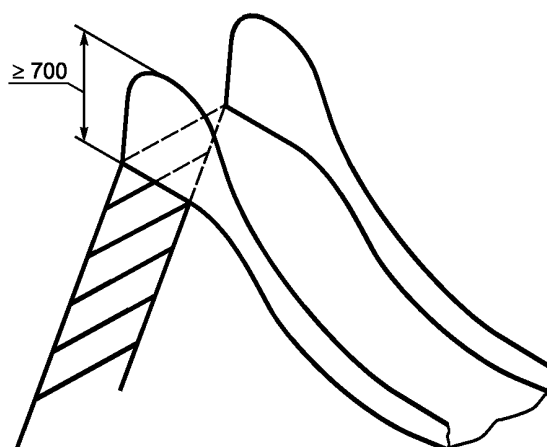
Рисунок 3 — Примеры стартового участка пристраиваемой и отдельно стоящей горок
