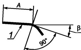
Рисунок 2 — Схема стартового участка
