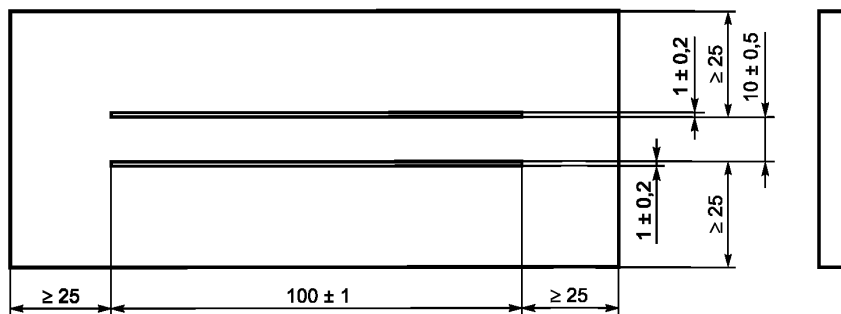
Рисунок 4 — Испытательный образец с электродами из проводящей краски
