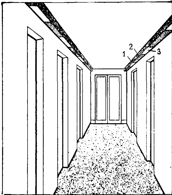
Рис. 71. Схема карнизного освещения коридора
