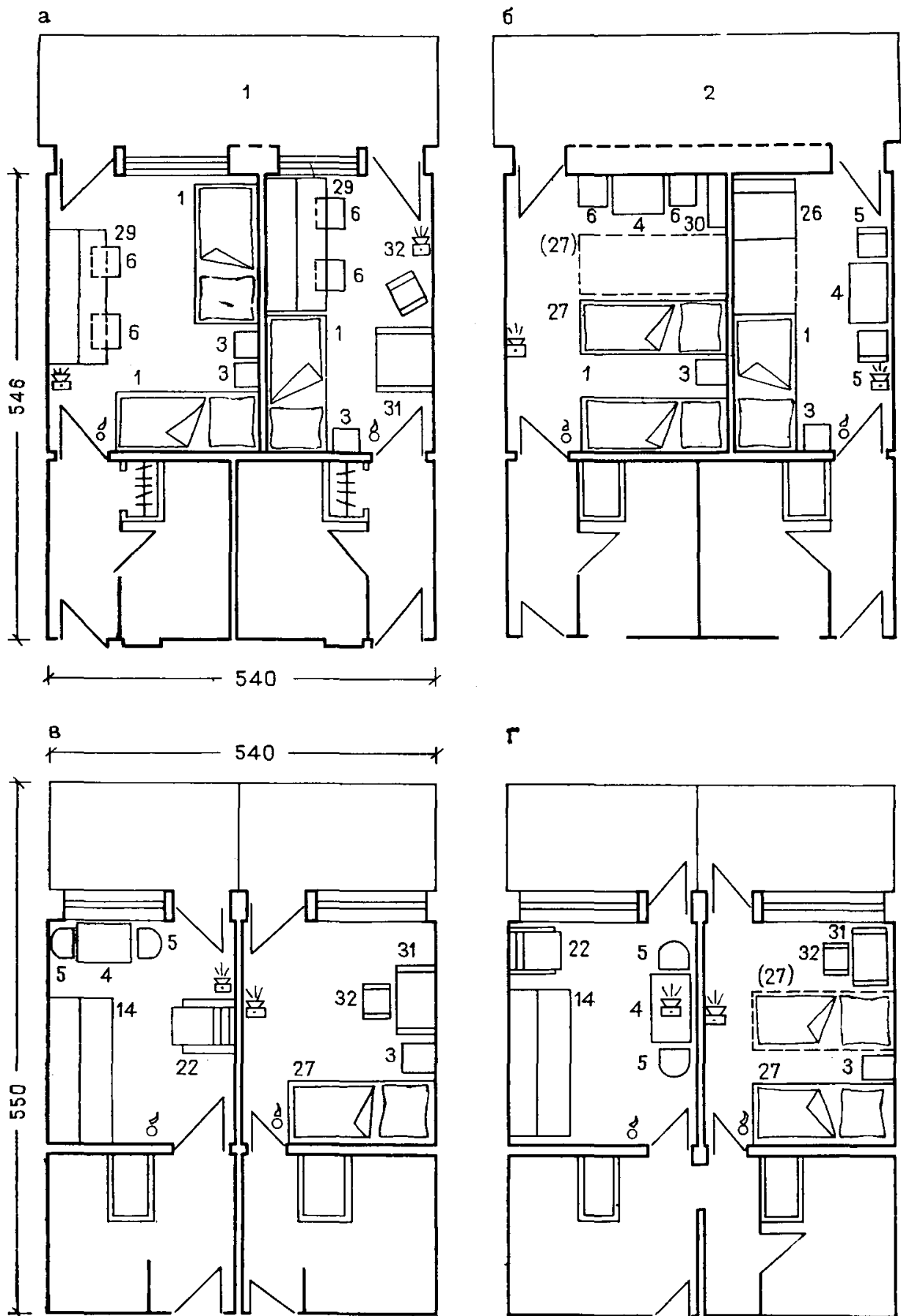
Рис. 8. Варианты использования одноместных и двухместных спальных ячеек для размещения семей с детьми (IV.1, IV.2, VII.1, VII.2)
