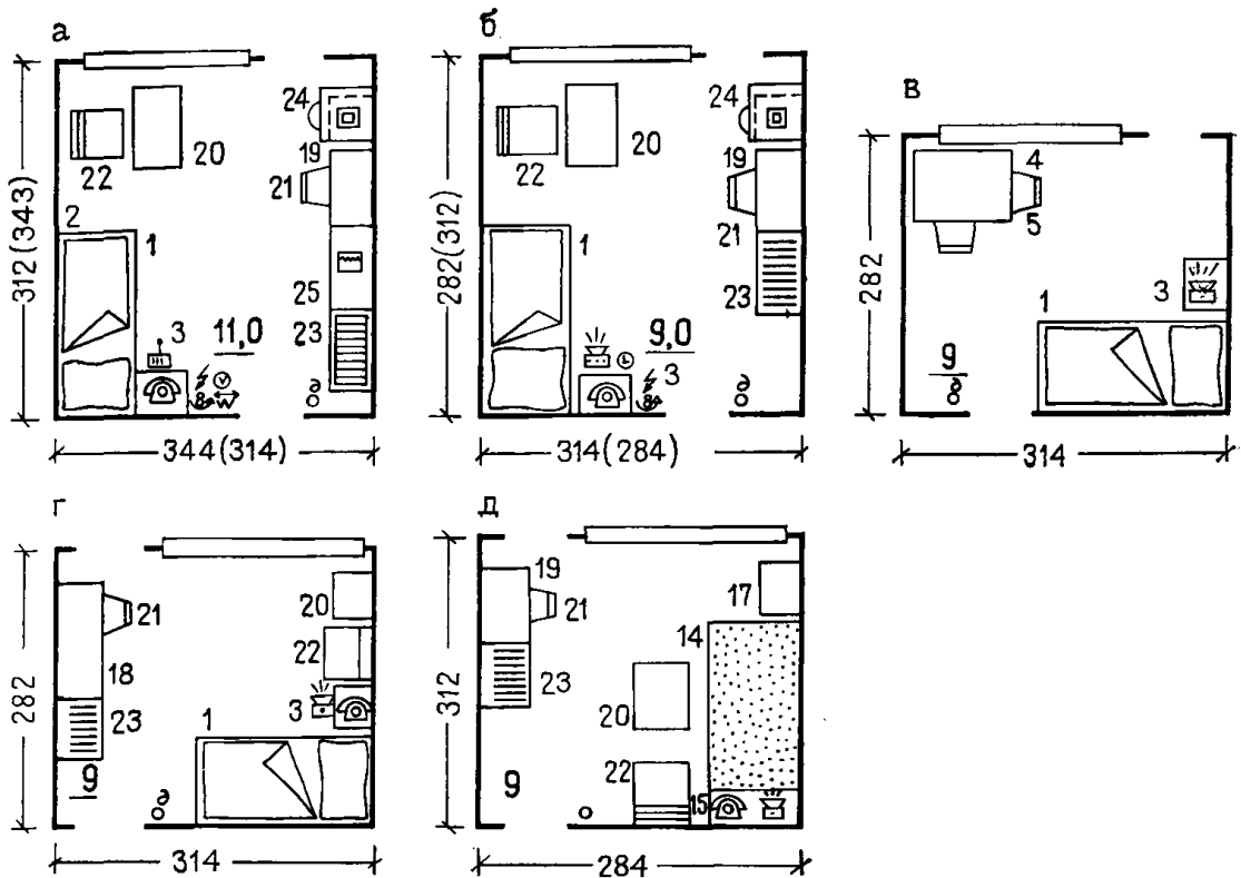
Рис. 1. Одноместные спальни. Расстановка мебели и оборудования
