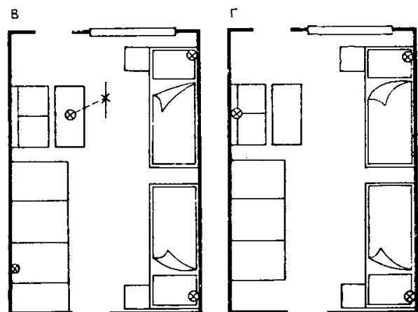
Рис. 51. Схемы решения искусственного освещения трехместных комнат в санаториях, домах отдыха, пансионатах, отелях и курортных гостиницах II разряда
