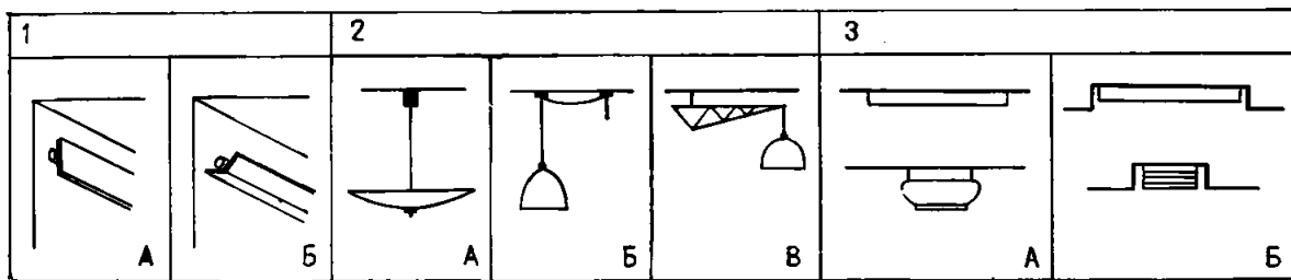
Рис. 40. Приемы общего освещения
