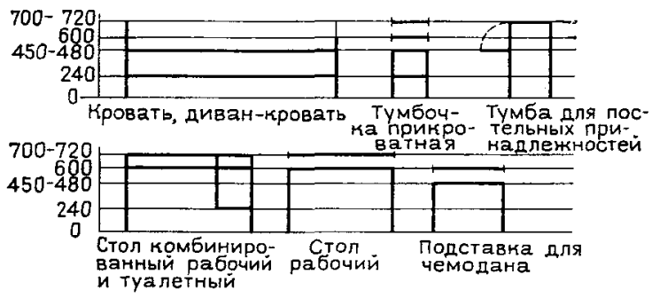
Рис. 14. Унификация размеров основных горизонтальных членений мебели
