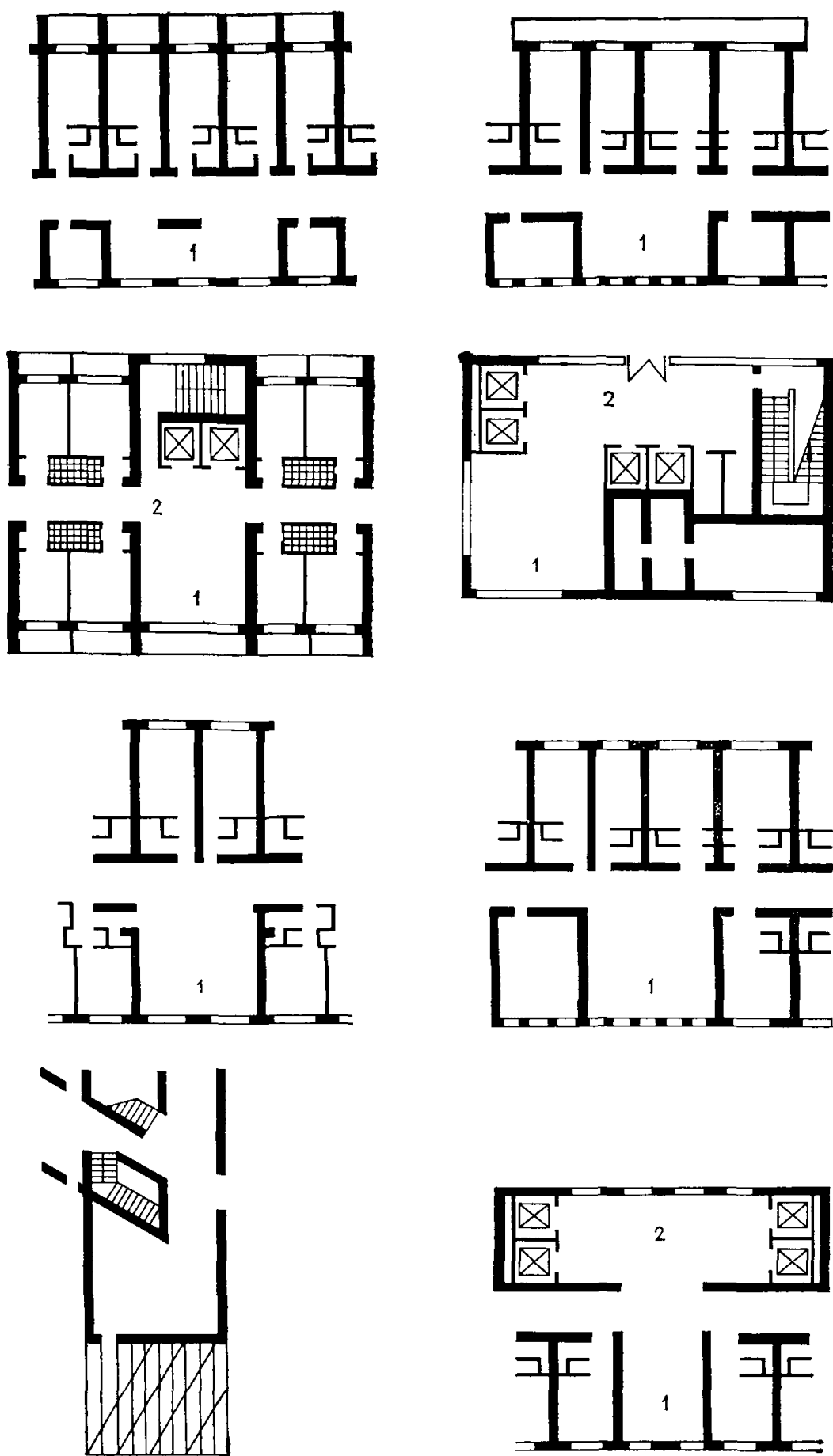
Рис. 63. Схемы планировки гостиных в спальнях корпусах 1 — гостиная; 2 — холл лифтовый
