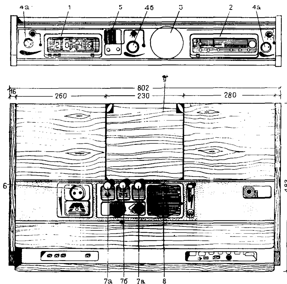
Рис. 27. Блок со встроенным оборудованием для спальных комнат. Экспериментальный образец НПО ГАУЯ ЛатвССР
