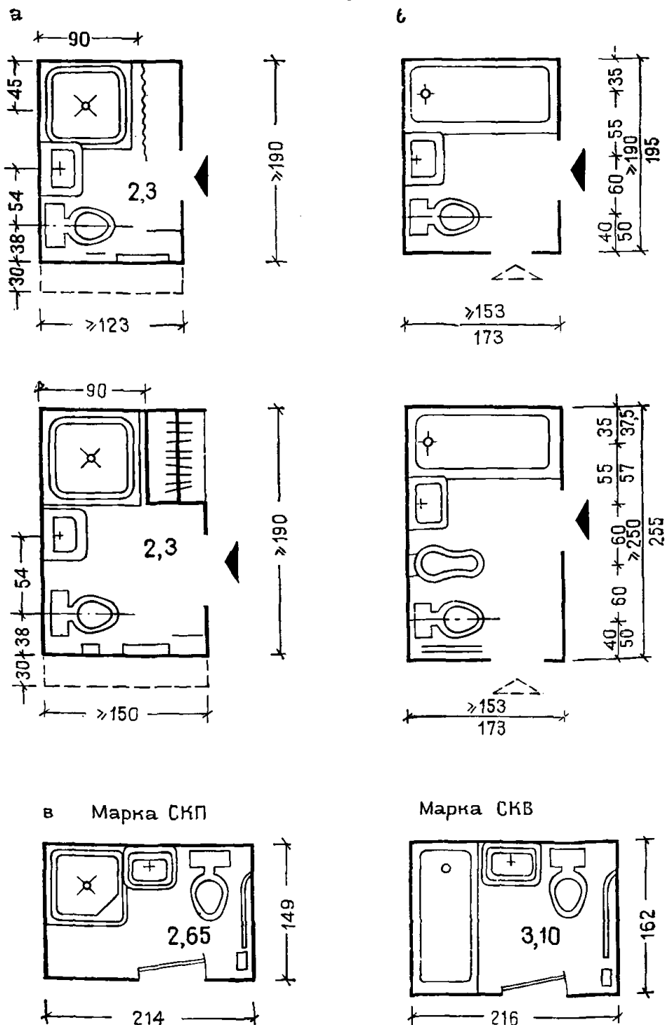
Рис. 57. Размещение оборудования в санузлах спальных ячеек
