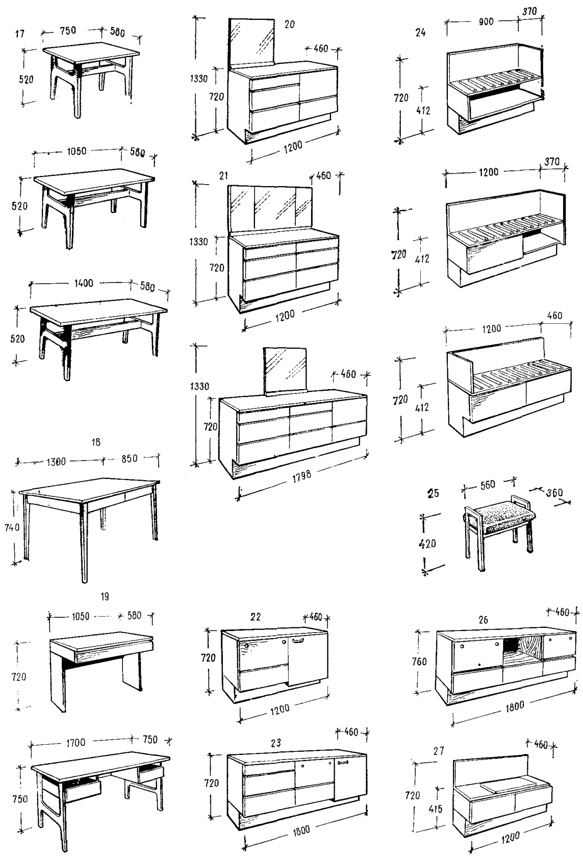
Рис. 32. Набор мебели для спальных комнат санаториев, домов отдыха и номеров гостиниц. Проект ВПКТИ мебели ОН-103-00, индекс ОН-5-456/1-11к Схема отдельных изделий набора мебели
