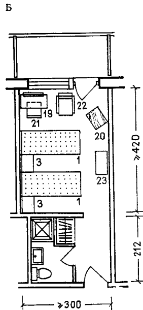
Рис. 22. Система мебели из отдельно стоящих блокируемых изделий (кровать типа 2 или 3)
