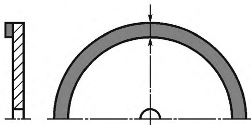
Рисунок 2 — Ширина диска с алмазным покрытием
