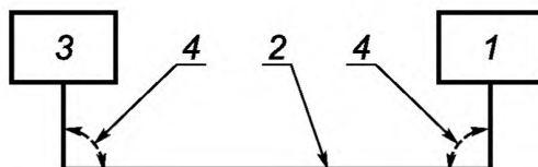
1 — ИО; 2 — испытуемые провода; 3 — имитатор нагрузки; 4 — угол (90^{+45}_0)^\circ
