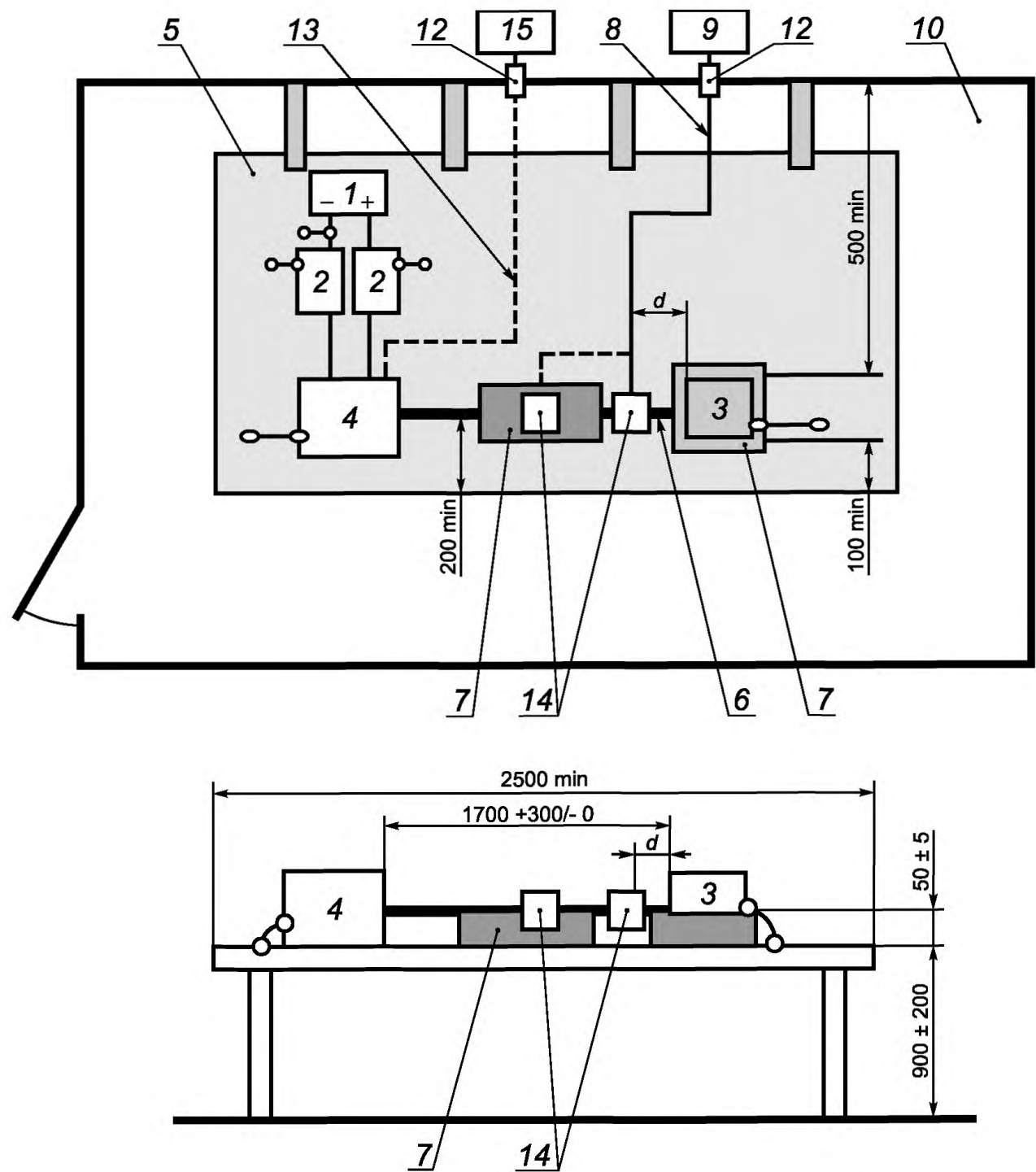
1 — источник питания; 2 — эквивалент сети; 3 — ИО (корпус заземлен, если это требуется в плане испытания); 4 — имитатор нагрузки (размещение и заземление в соответствии с [2]); 5 — пластина заземления; 6 — жгут проводов; 7 — подставка из материала с низкой относительной диэлектрической проницаемостью \epsilon_r \leq 1,4 ; 8 — коаксиальный кабель высокого качества, например, с двойным экранированием, 50 Ом; 9 — измерительное устройство; 10 — экранированное помещение; 12 — проходной разъем; 13 — волоконный световод; 14 — пробник тока (представлен в двух позициях); 15 — система мониторинга и моделирования; d — расстояние от ИО до ближайшей позиции пробника
