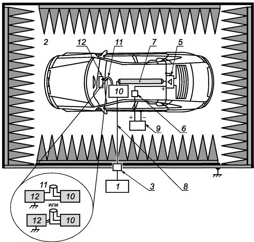
1 — измерительное устройство; 2 — БЭК; 3 — проходной разъем; 5 — усилитель антенны транспортного средства; 6 — силовой штекер усилителя питания; 7 — коаксиальный кабель антенны; 8 — коаксиальный кабель высокого качества с двойным экранированием 50 Ом; 9 — внешний аккумулятор 12 В; 10 — блок согласования; 11 — модифицированный коаксиальный «Т» разъем или короткое соединение с корпусом бортовой радиосистемы; 12 — корпус бортовой радиосистемы
