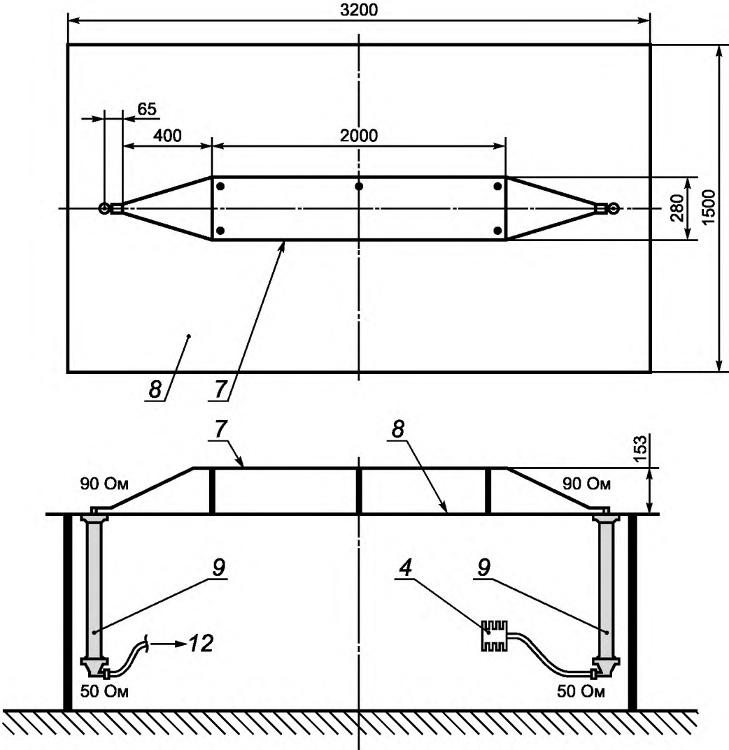
4 — нагрузка 50 Ом; 7 — перегородка; 8 — пластина заземления; 9 — согласующее устройство; 12 — измерительное устройство
