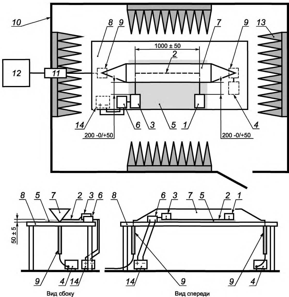
1 — ИО; 2 — испытуемые провода; 3 — имитатор нагрузки; 4 — нагрузка 50 Ом (размещение по выбору); 5 — подставка из материала с низкой относительной диэлектрической проницаемостью \epsilon_r \leq 1,4 ; 6 — эквивалент сети (ЭС); 7 — перегородка; 8 — пластина заземления; 9 — согласующее устройство (если необходимо); 10 — стенка экранированной комнаты; 11 — проходной разъем; 12 — измерительное устройство; 13 — поглотители (если необходимы); 14 — источник питания
