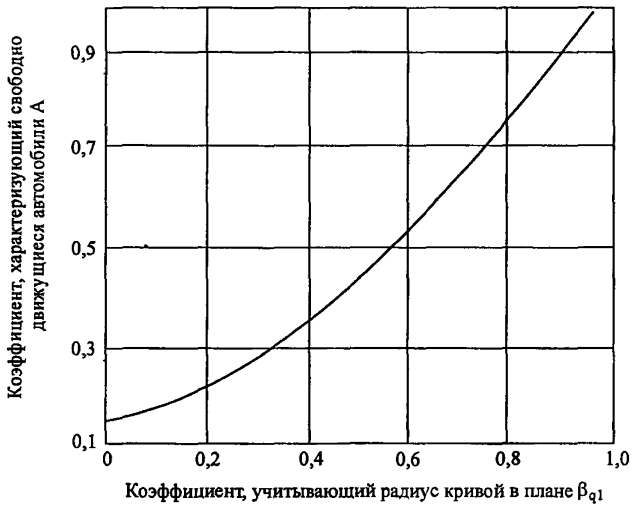
Рисунок 4 – Зависимость между коэффициентами A и \beta_1
