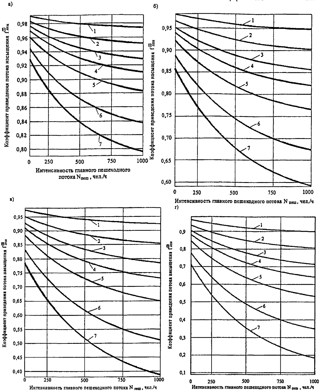
а – доля левоповоротного потока P_{ЛП} = 0,25 ; б – то же, P_{ЛП} = 0,5 ; – в – то же, P_{ЛП} = 0,75 ; г – то же, P_{ЛП} = 1 ; 1 – транспортный поток противоположного направления N_{пол} = 1000 прив.ед./ч на полосу; 2 – то же, N_{пол} = 600 прив.ед./ч; 3 – то же, N_{пол} = 400 прив.ед./ч; 4 – то же, N_{пол} = 300 прив.ед./ч; 5 – то же, N_{пол} = 200 прив.ед./ч; 6 – то же, N_{пол} = 100 прив.ед./ч; 7 – то же, N_{пол} = 0 .
