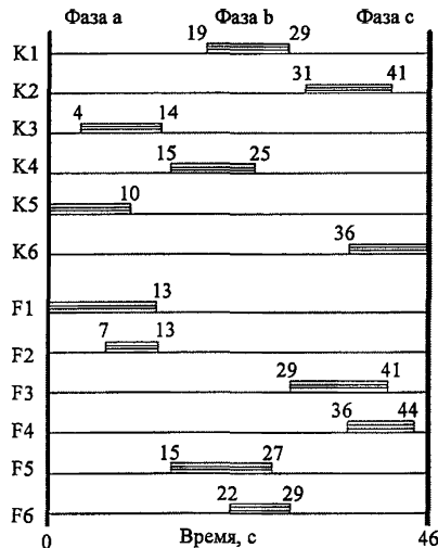
Рисунок И.3 – План светофорной сигнализации для пересечения, представленного на рисунке И.1 (цифрами показано время зеленого сигнала)
