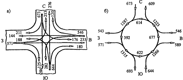
а – распределение по направлениям; б – распределение по кольцу Рисунок Ж.1 – Картограмма интенсивности движения
