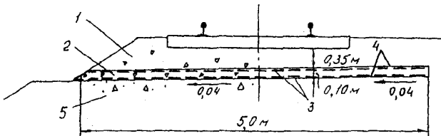
Рис. 4. Схема многослойного покрытия из георешетки (сварной сетки) и нетканого материала иглопробивного производства под балластным слоем: 1 - щебень в балластном слое; 2 - щебень между слоями георешетки и нетканого материала; 3 - георешетка; 4 - нетканый материал; 5 - загрязненный балласт
