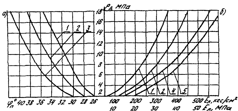
Рис. 2. Графики зависимости условного динамического сопротивления \rho_{\text{д}} от угла внутреннего трения \varphi_n для любой глубины (а) и модуля деформации E_n до глубины 6 м (б) для песчаных грунтов: 1 - пылеватых; 2 - мелких; 3 - крупных и средней крупности; 4 - средней крупности; 5 - крупных
