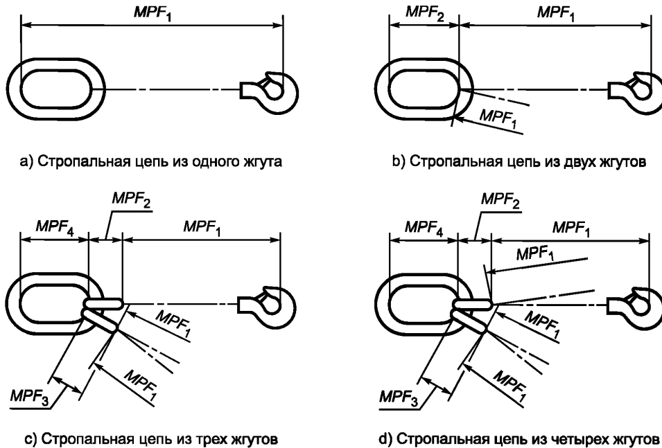
Рисунок 6 — Испытательные участки стропальных цепей
