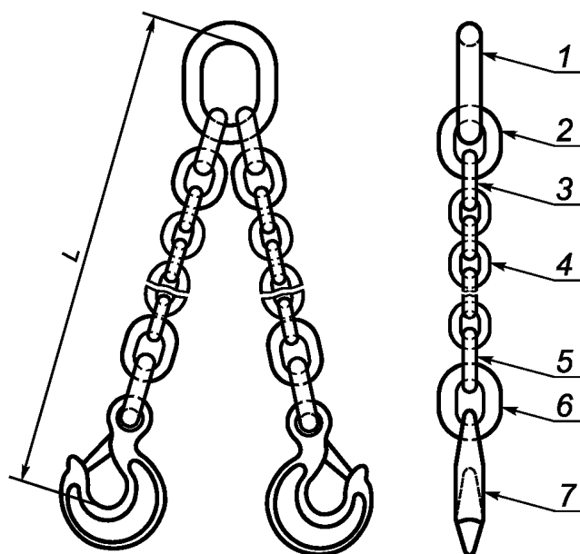
Рисунок 1 — Стропальные цепи из одного жгута
