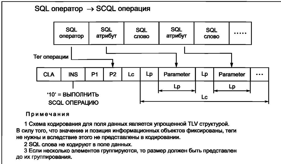
Рисунок 9 — Принцип отображения оператора SQL на SCQL операции
