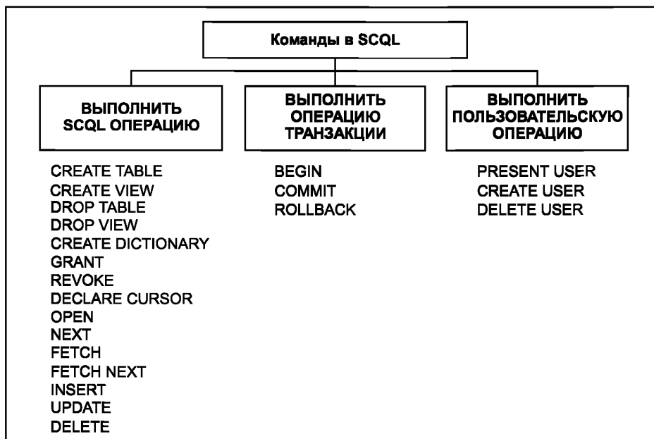
Рисунок 10 — Команды в SCQL
