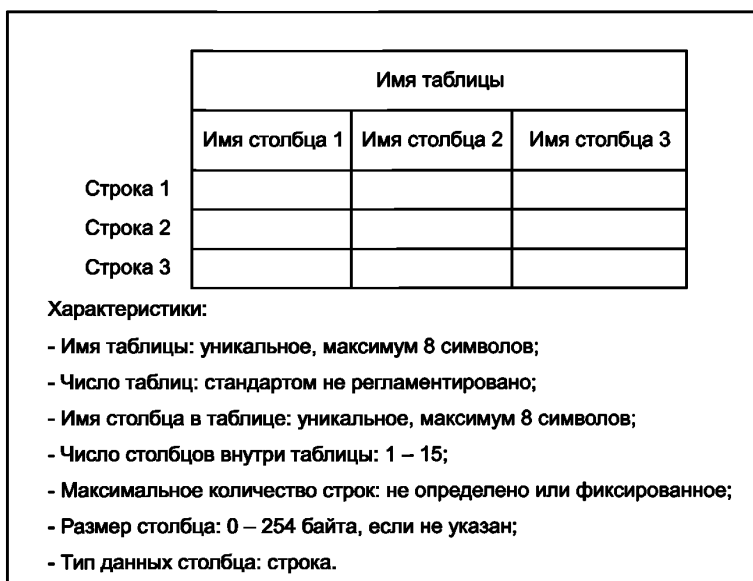
Рисунок 3 — Таблица SCQL (пример) и ее главные характеристики
