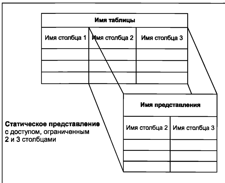
Рисунок 4 — Статическое представление SCQL (пример)
