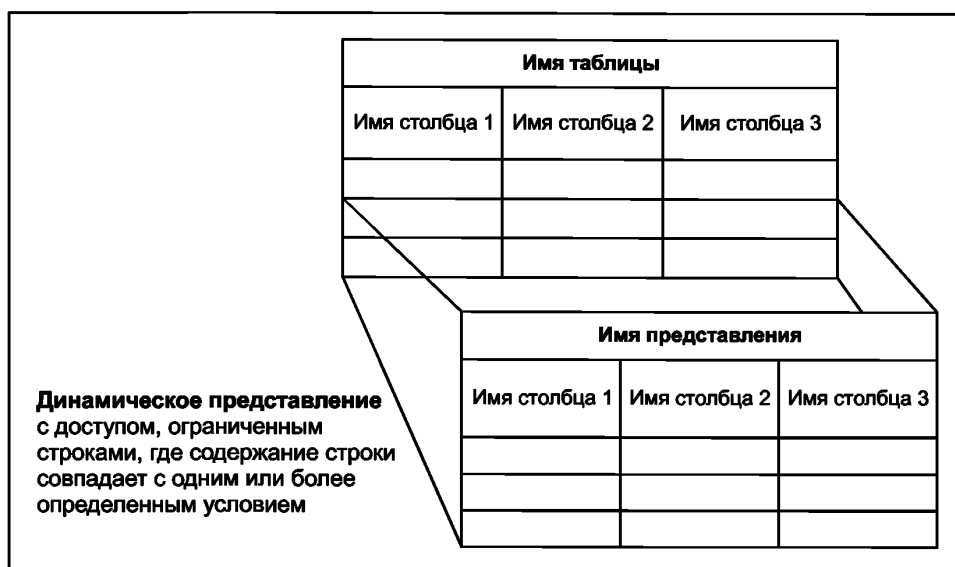
Рисунок 5 — Динамическое представление SCQL (пример)
