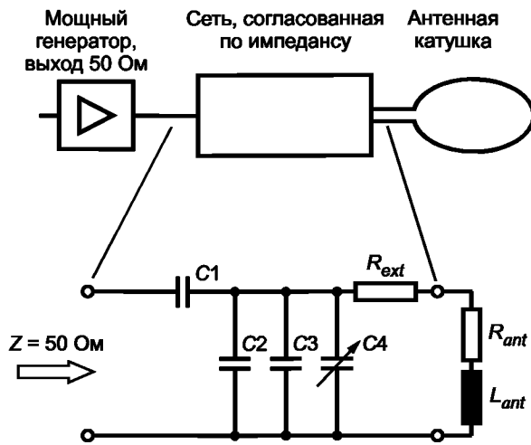
Рисунок А.3 — Сеть, согласованная по импедансу
