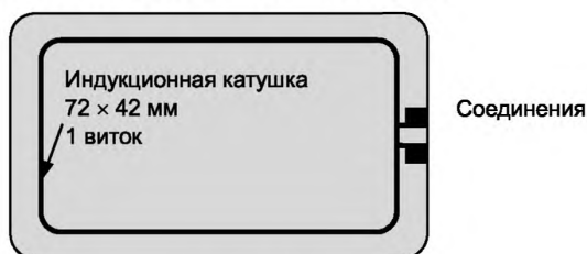
Рисунок 3 — Калибровочная катушка
