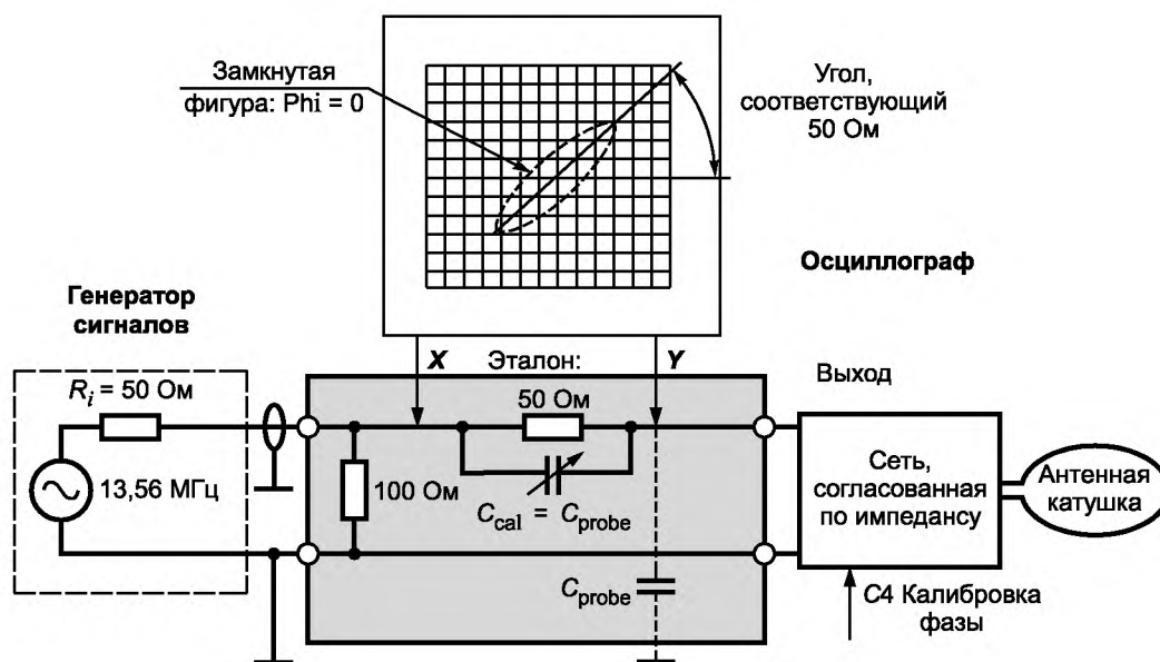
Рисунок В.2 — Схема настройки (этап 2)
