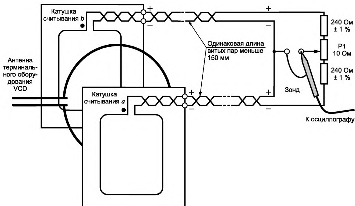
Рисунок 4 — Принципиальная схема испытательной установки
