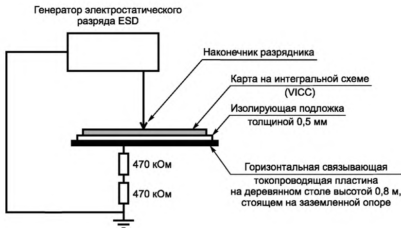
Рисунок 1 — Цепь испытания на воздействие статического электричества
