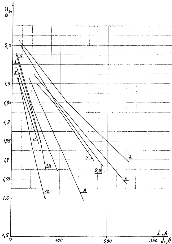
Рис. 2. Зависимость напряжения U_3 одной пары пластин аккумулятора от величины толчкового тока I_T для аккумуляторов типа GzOE и с намазными пластинами (Вольт-Амперные характеристики).
