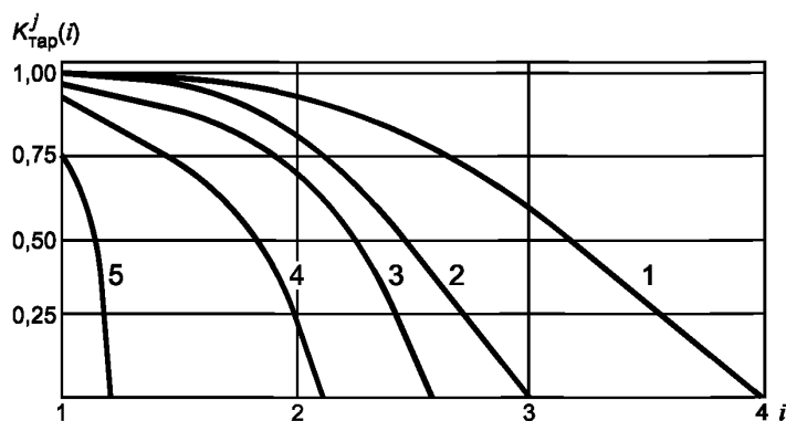
Рисунок 1 — Серия тарифовочных кривых K_{\text{тар}}^j(i)
