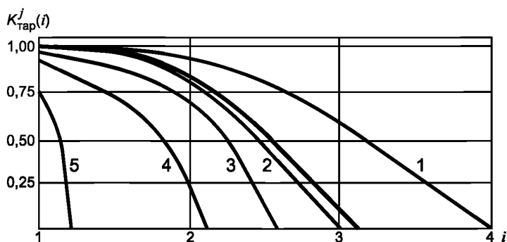
Рисунок 2 — Зависимость K(i) , нанесенная на серию тарифовочных кривых
