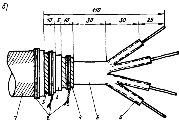
Рис.5. Схема разделки концов кабеля СМКПВК 1х4х1,2 и МКВБ 1х4х1,2:
