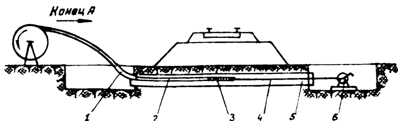
Рис. 10. Затягивание кабеля в трубу:
