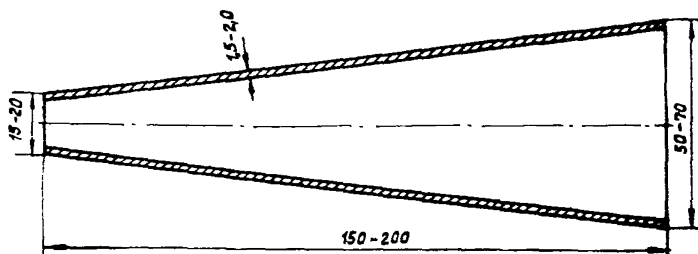
Рис.8. Защитный конус-воронка
