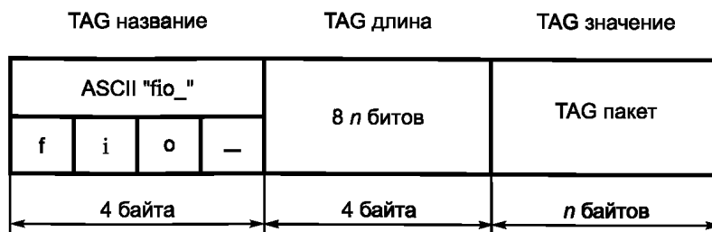
Рисунок Б.1 — Файл вход/выход
