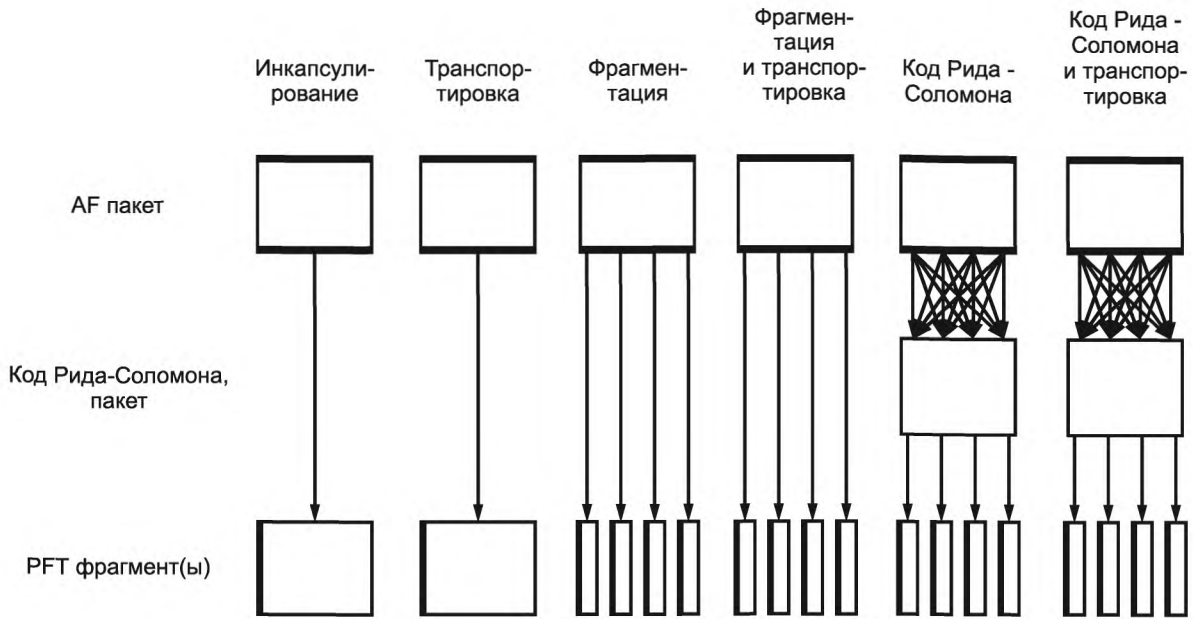
Рисунок 10 — Доступные опции с использованием уровня PFT
