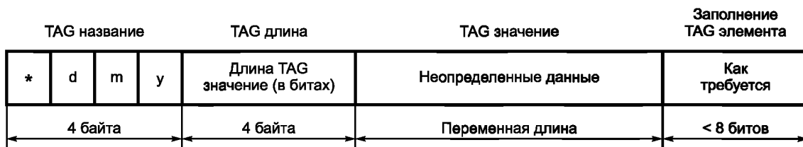
Рисунок 8 — Фиктивное заполнение TAG элемента
