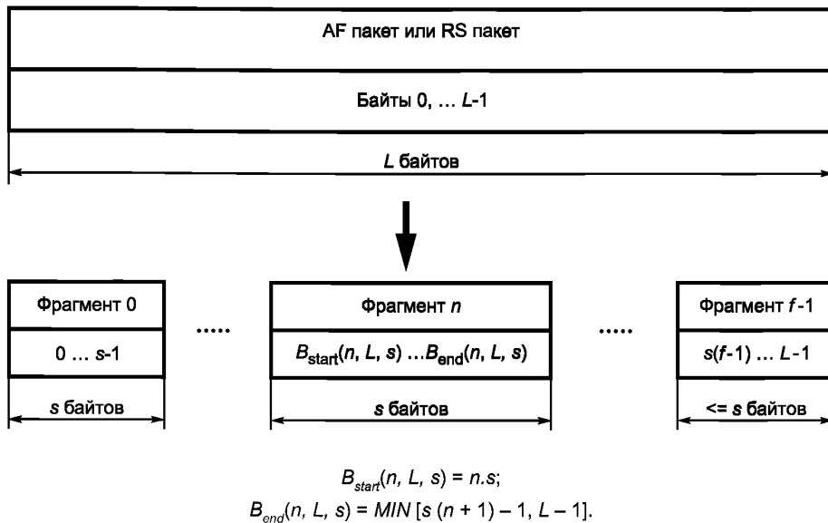
Рисунок 13 — Фрагментация AF или RS пакета
