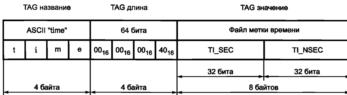
Рисунок Б.3 — Файл метки времени
