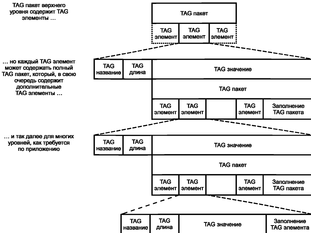
Рисунок 6 — Иерархические TAG элементы
