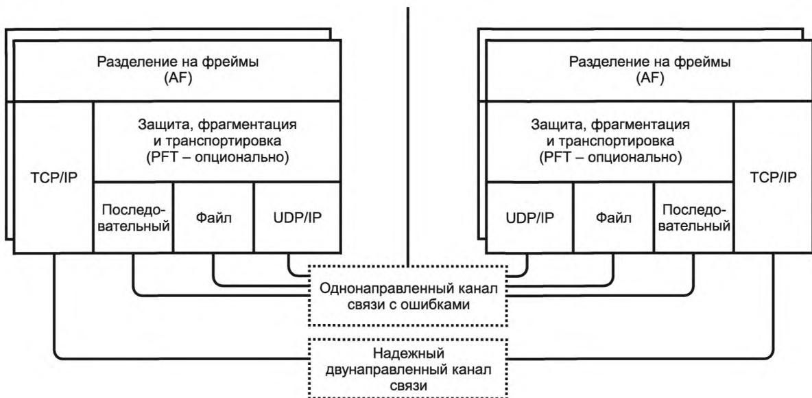
Рисунок 2 — Пример уровней связи DCP
