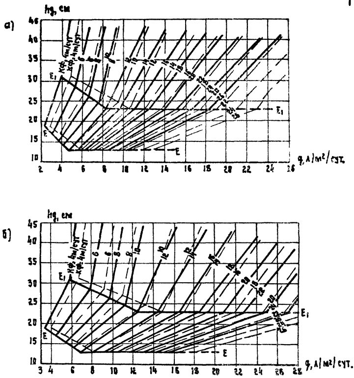
Рис. 22 График для определения толщины дренажного слоя при поперечном профиле дорожной одежды с индексом \Delta и пути фильтрации 11\text{ м} .
