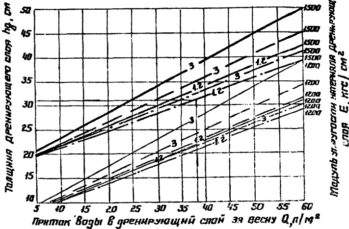
Рис. 5 График для определения толщины дренажного слоя основания h_d из крупного песка при поперечном профиле проезжей части с индексом B
