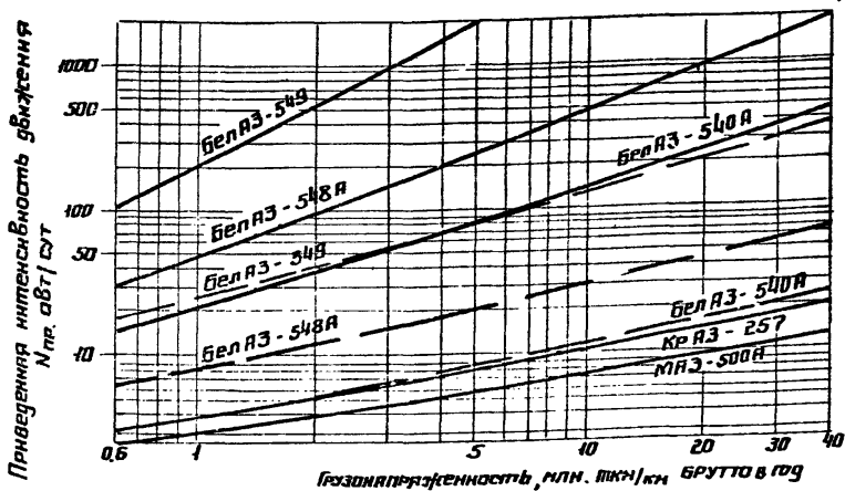
Рис 30 Номотриям для определения приведенной интенсивности движения к расчетному автомобилю БелАЗ-548. Обозначенная также, что и на Рис. 28
