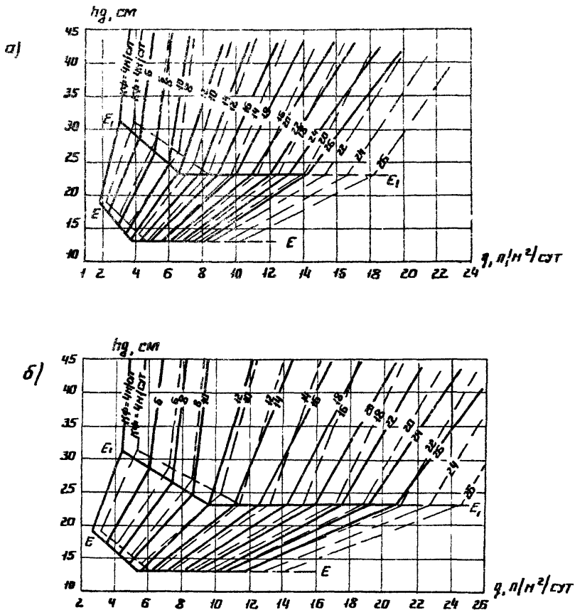
Рис 24 График для определения толщины дренажного слоя при поперечном профиле дорожной одежды с индексом J и путем фильтрации 13\text{ м} а - глубина ровника 25 см; б - глубина ровника 45 см. Обозначения те же, что и на рис. 7
