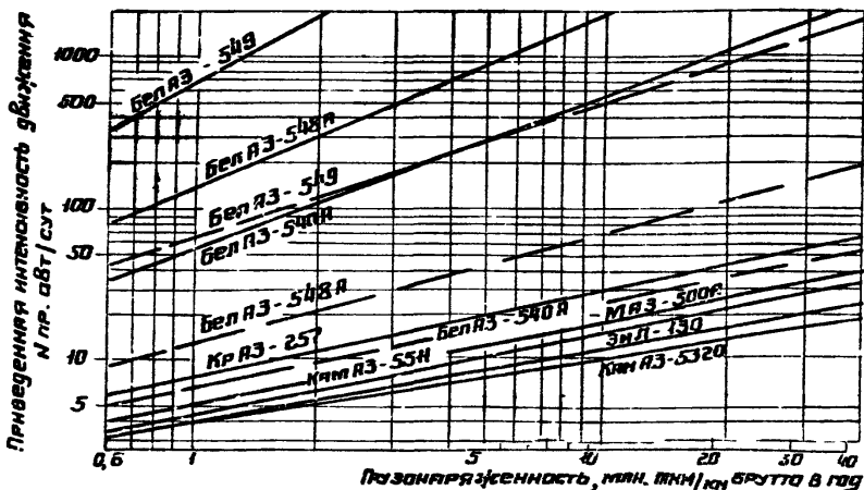
Рис. 29 Номаграмма для определения интенсивности движения к расчетному автомобилю БелАЗ - 540
