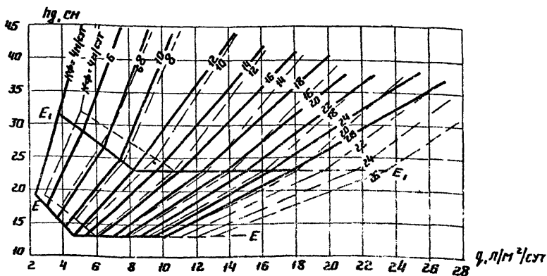
Рис. 12 График для определения толщины дренажного слоя при поперечном профиле дорожной одежды с индексом В и Г и пути фильтрации 9 м.
