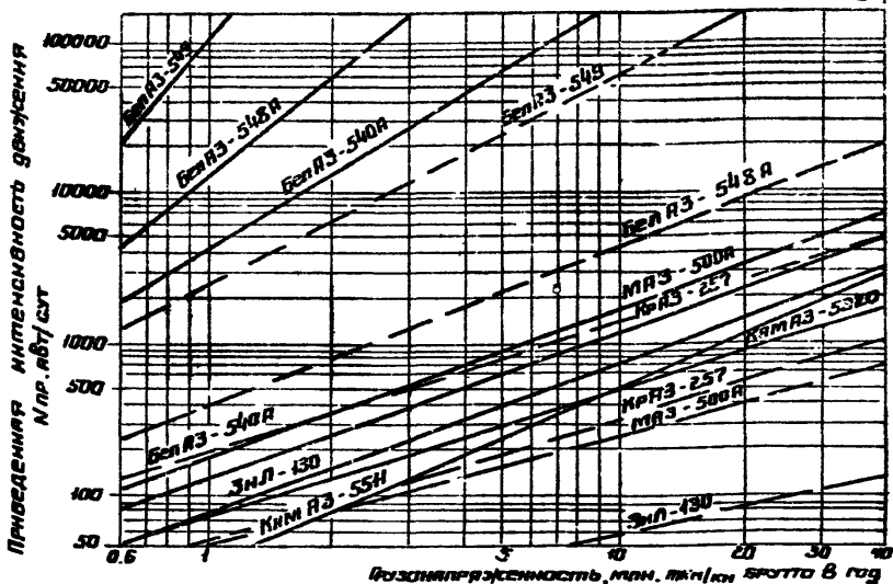
Рис. 28 Номаграмма для определения приведенной интенсивности движения к расчетному автомобилю группы А
