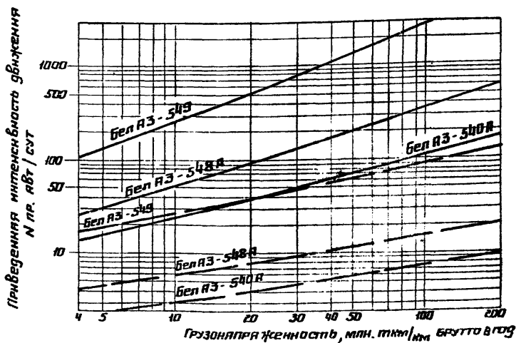
Рис 31 Номотриям для определения приведенной интенсивности движения к расчетному автомобилю БелАЗ-548 Обозначенная также, что и на Рис. 28
