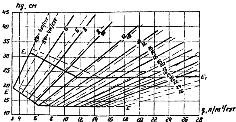
Рис. 10. График для определения толщины дренажного слоя при поперечном профиле дорожной одежды с индексами В и Г и пути фильтрации 7 м. Обозначения те же, что и на рис. 7
