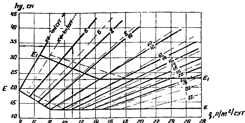
Рис. 9. График для определения толщины дренажного слоя при поперечном профиле дорожной одежды с индексами В и Г и пути фильтрации 6 м. Обозначения те же, что и на рис. 7
