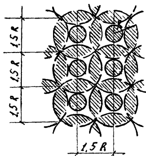
Схема перестановки вибраторов в рядовом порядке
