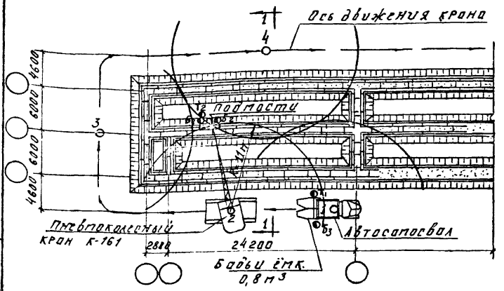
Схема бетонирования ленточных фундаментов с помощью стрелового крана
