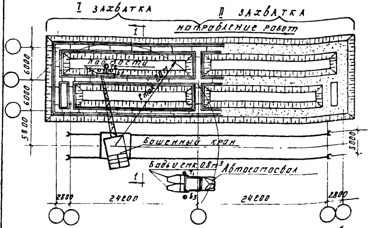
Схема бетонирования ленточных фундаментов с помощью башенного крана
