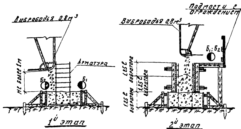
Бетонирование ленточных фундаментов в щитовой опалубке
