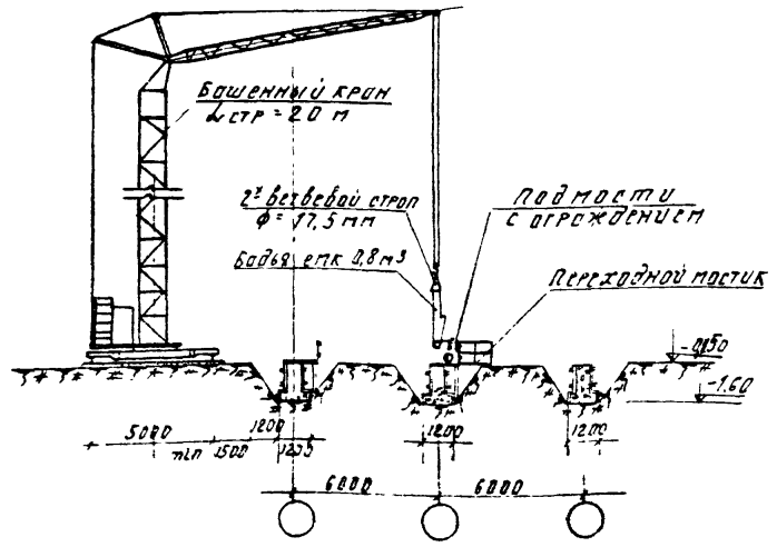
Разрез 1-1
