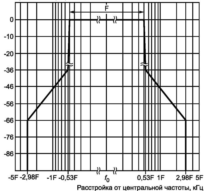
Рисунок 2 — Маска огибающей внеполосных радиоколечаний в логарифмических координатах
