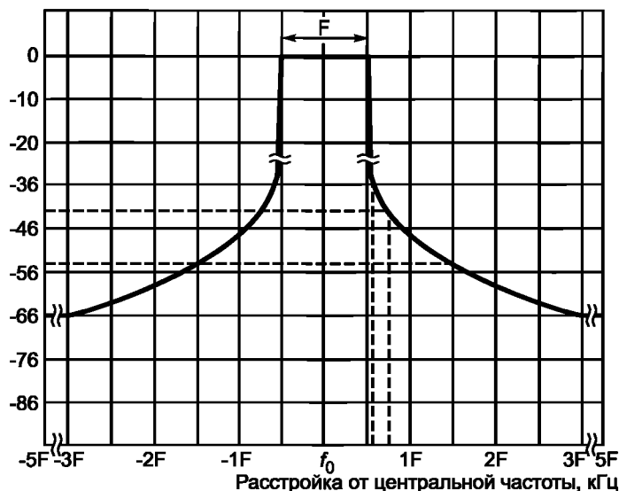
Рисунок 1 — Маска огибающей внеполосных радиоколечаний в линейных координатах
