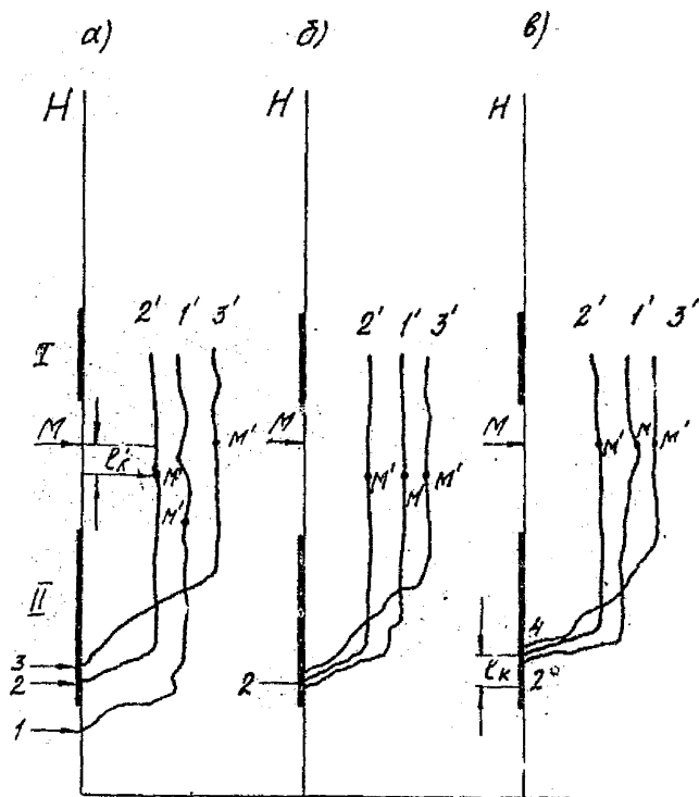
Рис.21. Коррекция профилей по глубине а) Некорректированные профили б) Профили, корректированные относительно друг друга в) Профили, корректированные относительно муфты II.
