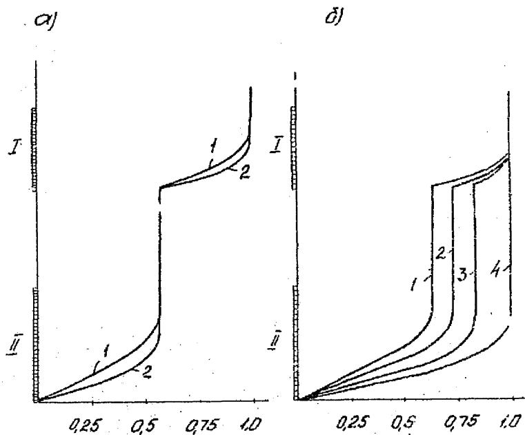
Рис. 28. Видны трансформация профилей притока в процессе эксплуатации
