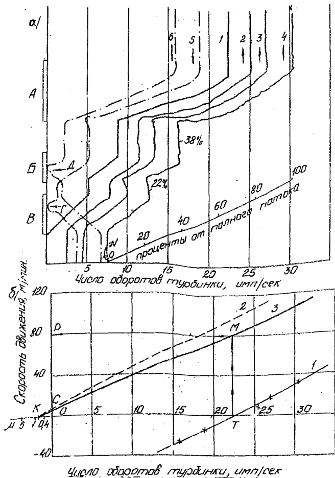
Рис. 19. Профили, полученные при непрерывной протяжке прибора с различными скоростями /калибровка "на месте".
