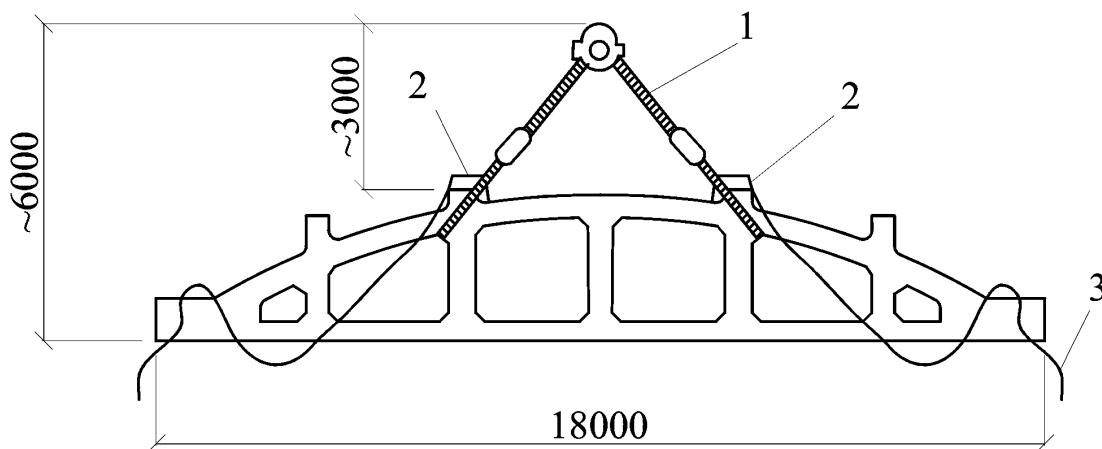
1 – строп; 2 – пружинный замок Пр8; 3 – канат для расстропки
