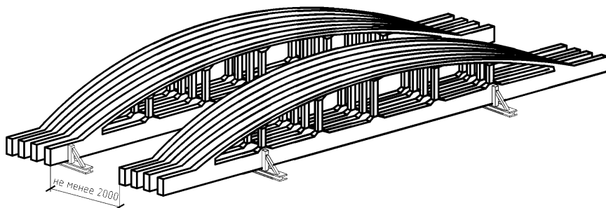
Рисунок 6 – Схема опирания при транспортировке и хранении ферм
