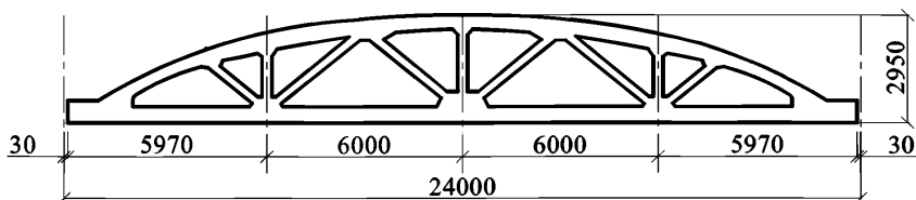
Рисунок 1 – Раскосная сегментная ферма
