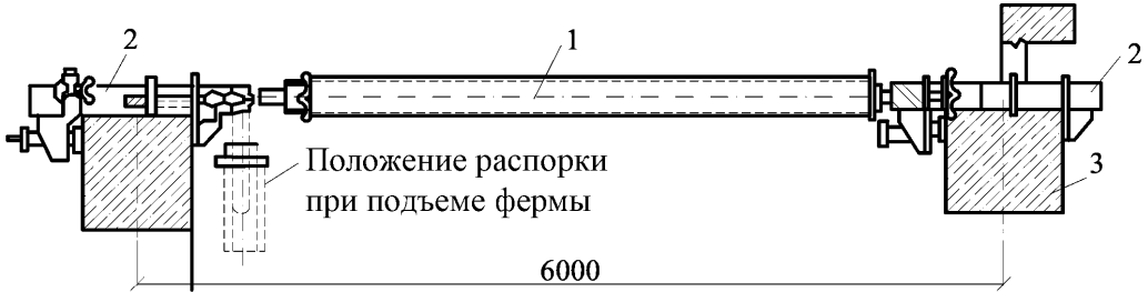
Рисунок 11 – Инвентарная распорка
