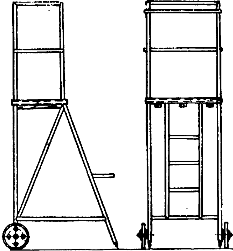
Рисунок 13 – Передвижная площадка монтажника
