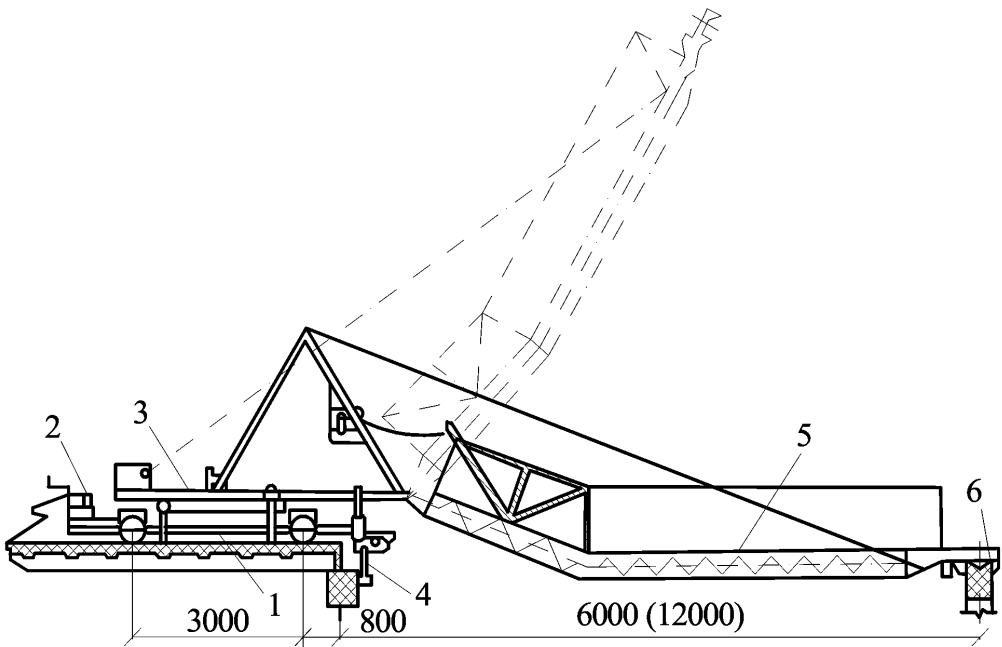
Рисунок 11 – Инвентарная распорка
