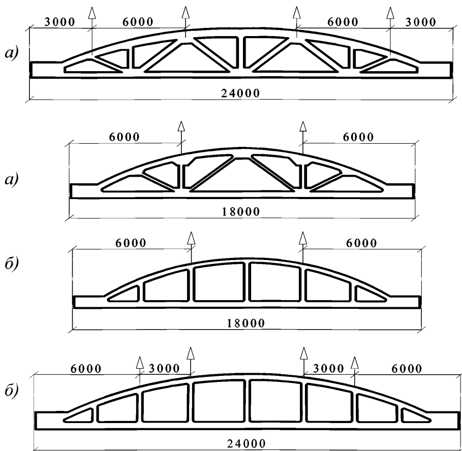
а) схема строповки раскосных ферм, б) схема строповки безраскосных ферм
