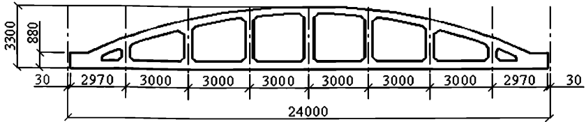
Рисунок 2 – Безраскосная ферма
