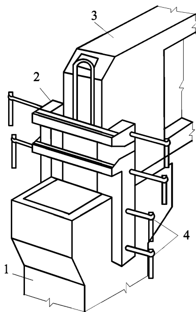
1 – колонна; 2 – рама кондуктора; 3 – ферма; 4 – зажимные винты
