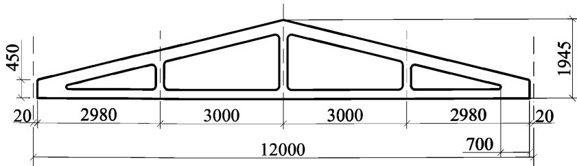
Рисунок 3 – Безраскосная треугольная ферма
