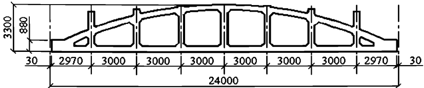
Рисунок 4 – Безраскосная ферма для покрытий с малоуклонной кровлей
