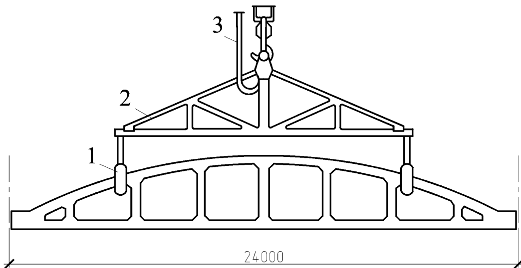
1 – захват; 2 – жесткая траверса; 3 – кабель
