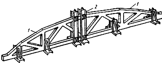
1 – полуферма; 2 — парные стойки
